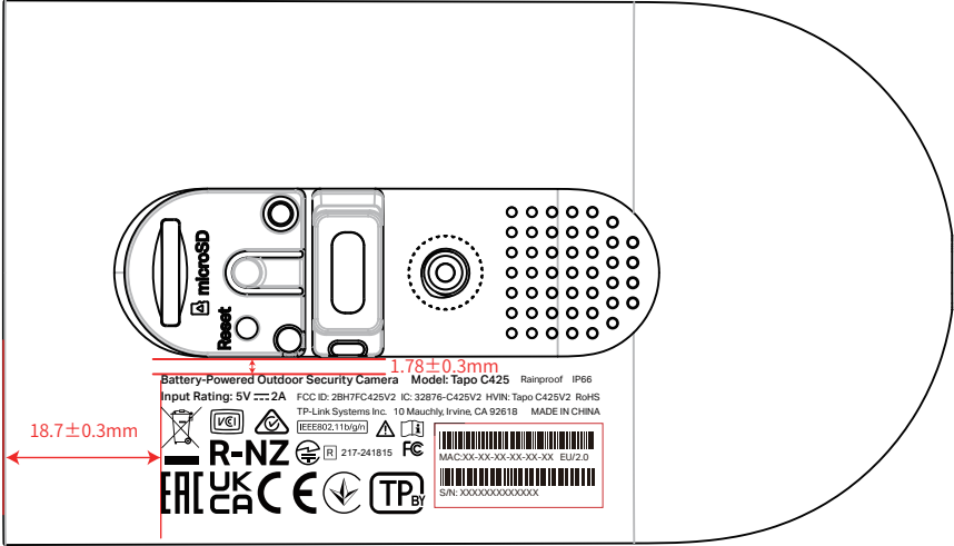
尺寸图
