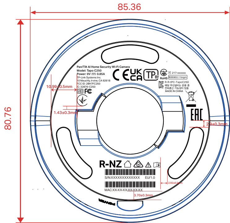
尺寸图
