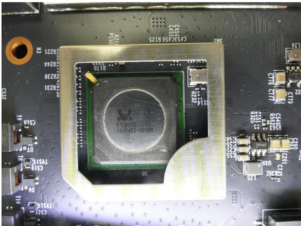
(37) EUT Photo
