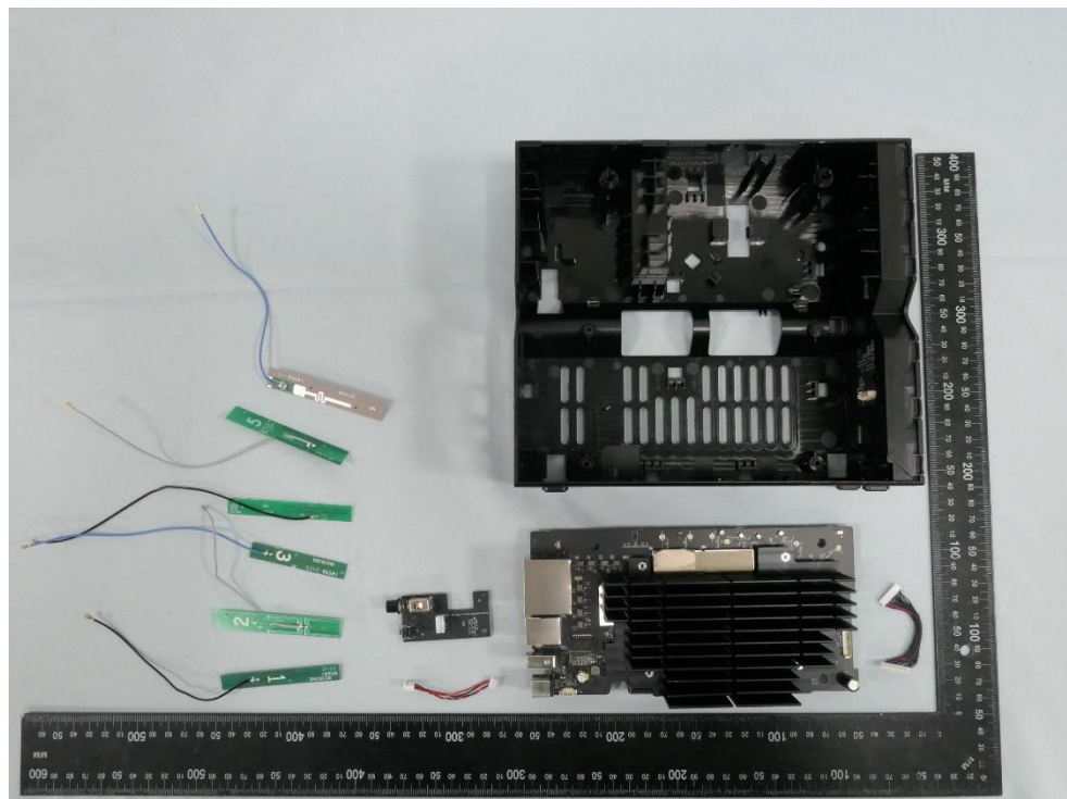
(19) EUT Photo
