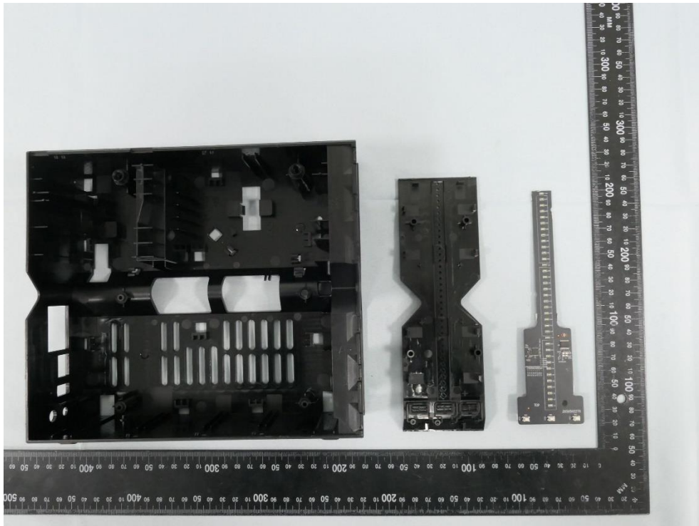
(50) EUT Photo
