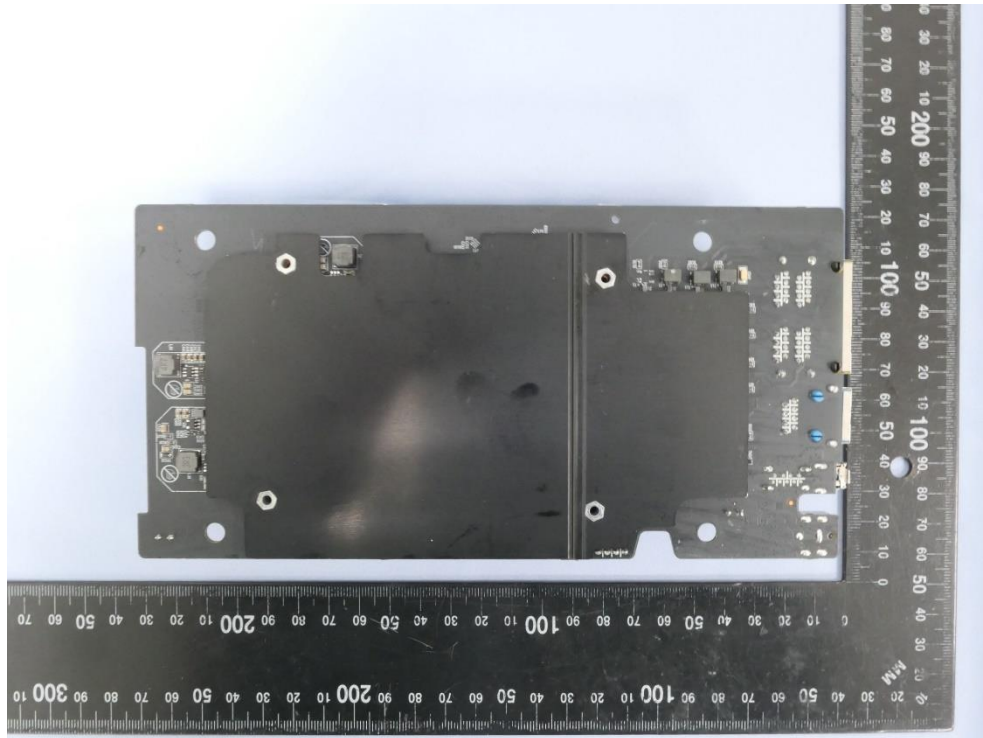
(46) EUT Photo
