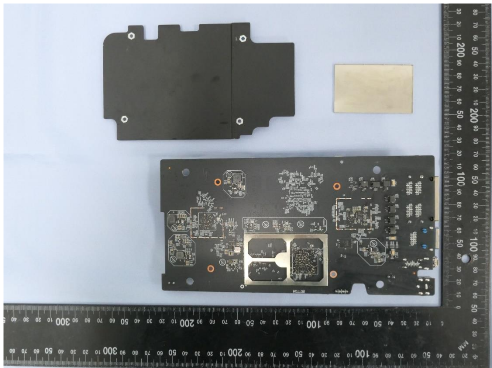
(47) EUT Photo
