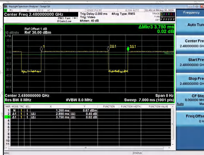
NTNV-2DH5-Ant1-2480
