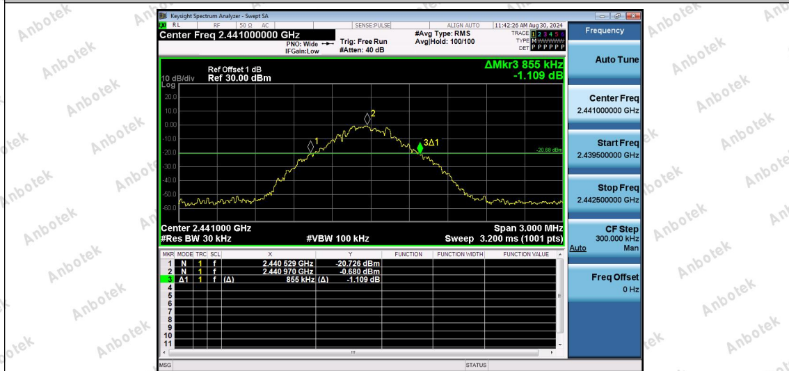
2.4G-Ant1-2441
