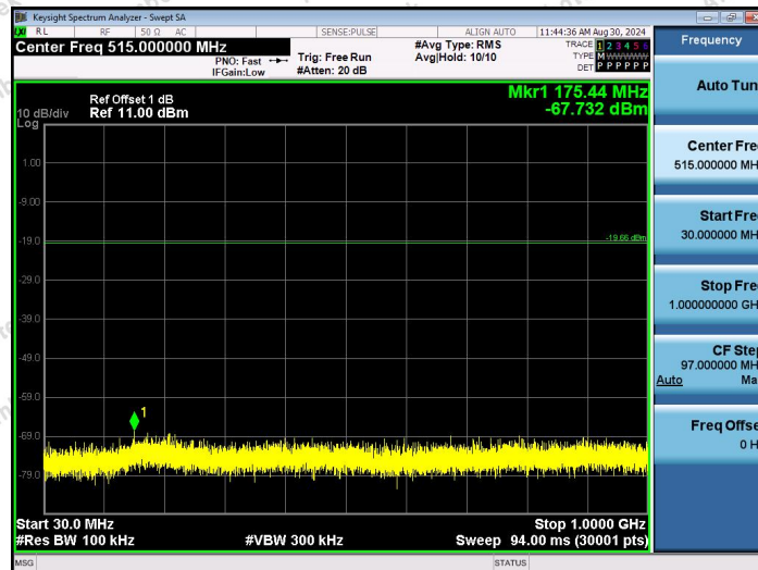
2.4G-Ant1-2480-30~1000-PASS
