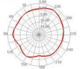
5850.000MHz E2
