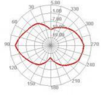
5850.000MHz H
