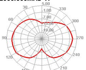
2500.000MHz H
