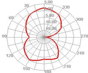
2450.000MHz E1
