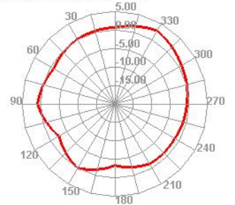
5850.000MHz E2
