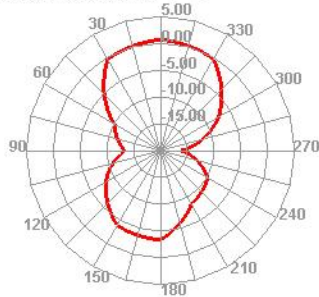
5850.000MHz E1
