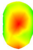
2400.000MHz E1
