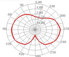
2450.000MHz H
