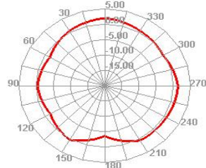
2450.000MHz E2
