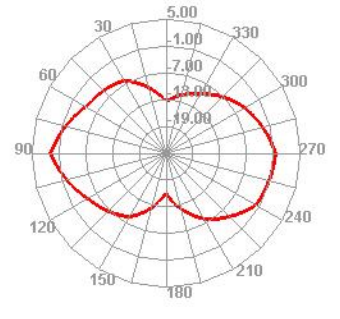
5850.000MHz H
