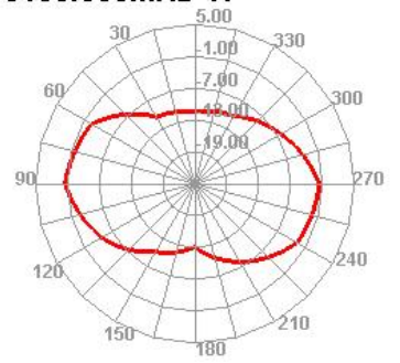
5150.000MHz H
