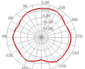
2500.000MHz E2
