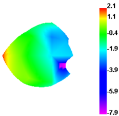
2400.000MHz
