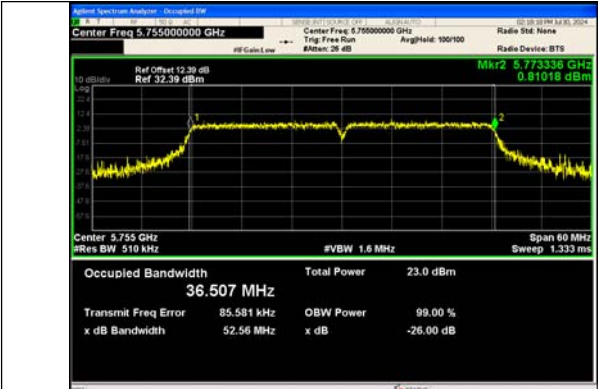
IEEE 802.11n_Channel 151_40MHz_Antenna 0
