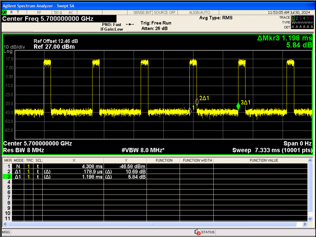
IEEE 802.11a 20MHz_Channel 140
