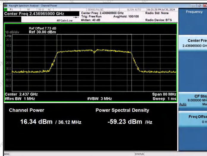
11AX40MIMO-Ant1-2437-PASS
