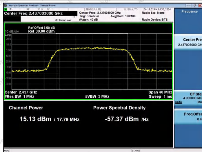
11AX20MIMO-Ant1-2437-PASS
