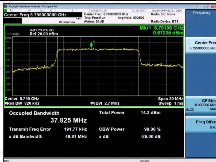
11AX40MIMO-Ant2-5795
