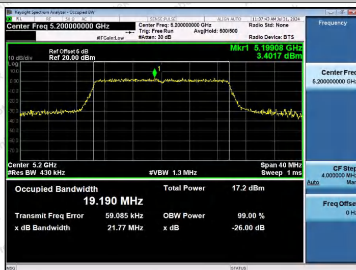
11AX20MIMO-Ant2-5200
