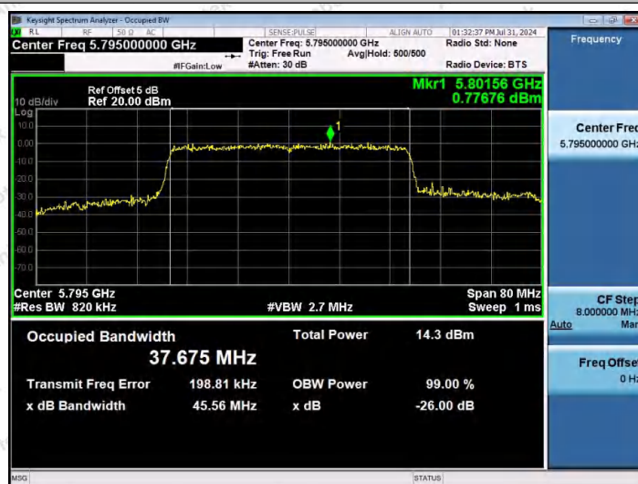
11AX40MIMO-Ant1-5795
