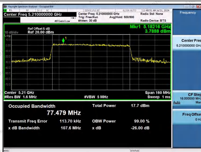
11AX80MIMO-Ant1-5210
