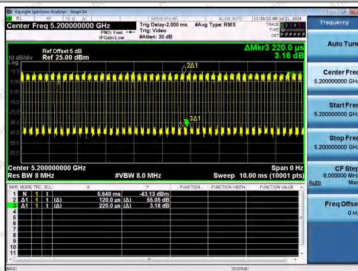
NTNV-11AX20MIMO-Ant1-5200
