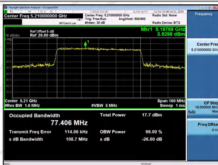
11AX80MIMO-Ant2-5210
