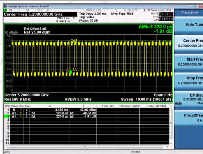
NTNV-11AX20MIMO-Ant2-5200
