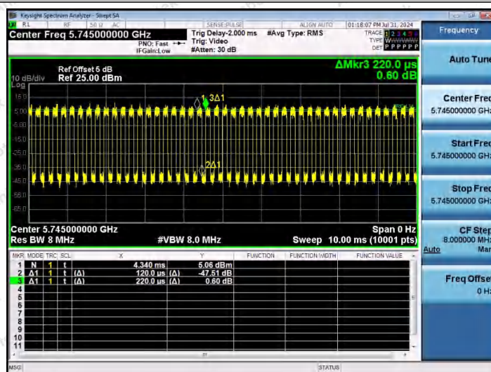
NTNV-11AX20MIMO-Ant1-5745
