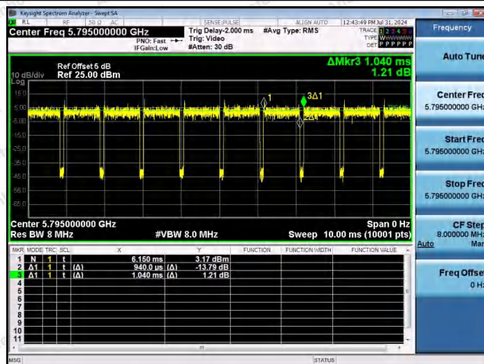
NTNV-11N40MIMO-Ant1-5795
