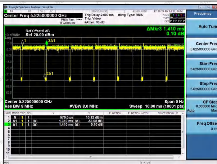
NTNV-11N20MIMO-Ant1-5825
