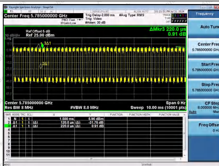
NTNV-11AX20MIMO-Ant1-5785
