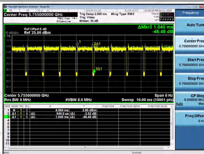
NTNV-11N40MIMO-Ant1-5755
