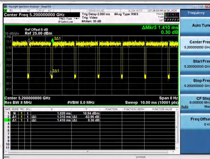
NTNV-11N20MIMO-Ant1-5200
