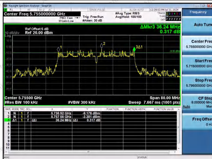
11N40MIMO-Ant1-5755-PASS
