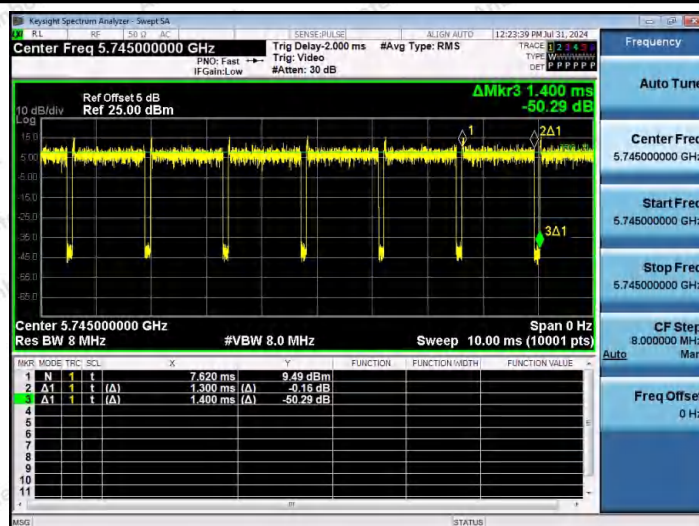
NTNV-11N20MIMO-Ant1-5745
