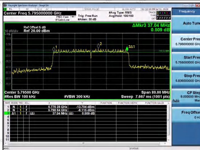
11AX40MIMO-Ant1-5795-PASS
