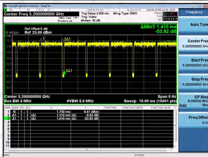
NTNV-11AC20MIMO-Ant1-5200
