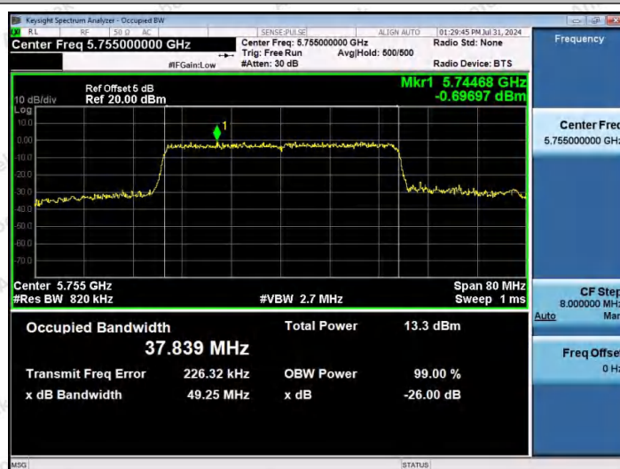
11AX40MIMO-Ant2-5755
