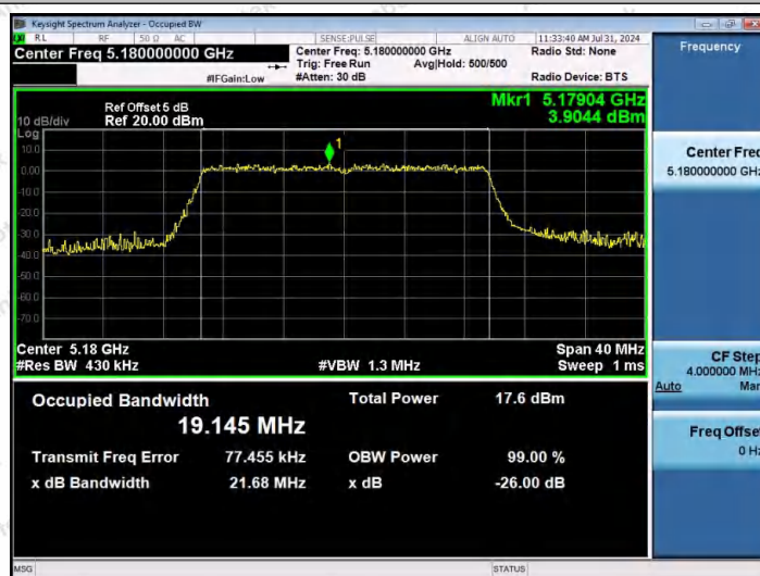
11AX20MIMO-Ant1-5180
