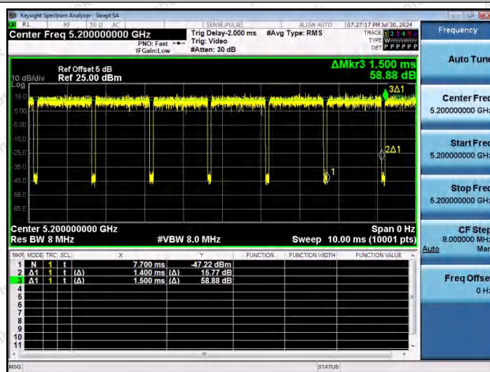
NTNV-11A-Ant1-5200
