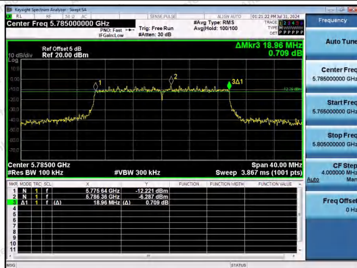
11AX20MIMO-Ant1-5785-PASS
