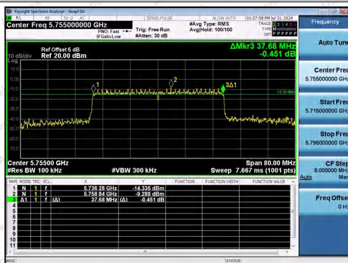
11AX40MIMO-Ant1-5755-PASS
