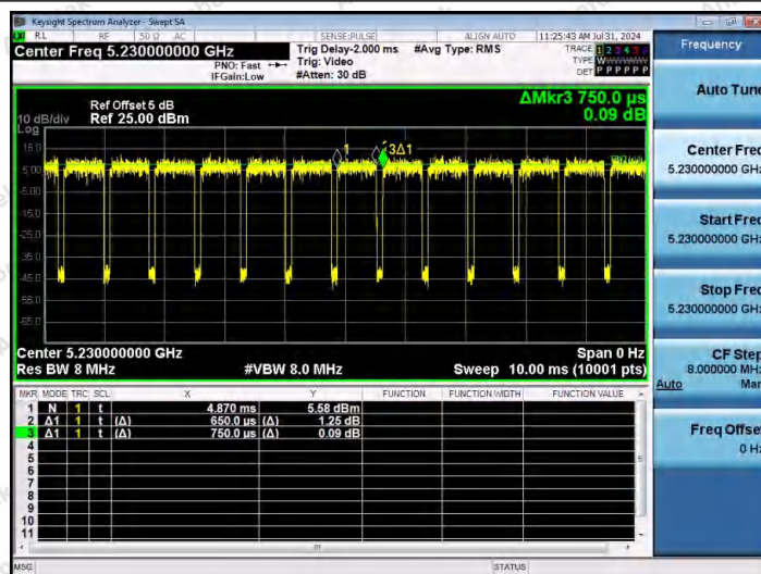
NTNV-11AC40MIMO-Ant1-5230
