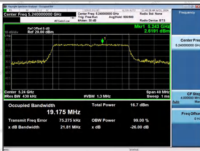
11AX20MIMO-Ant2-5240
