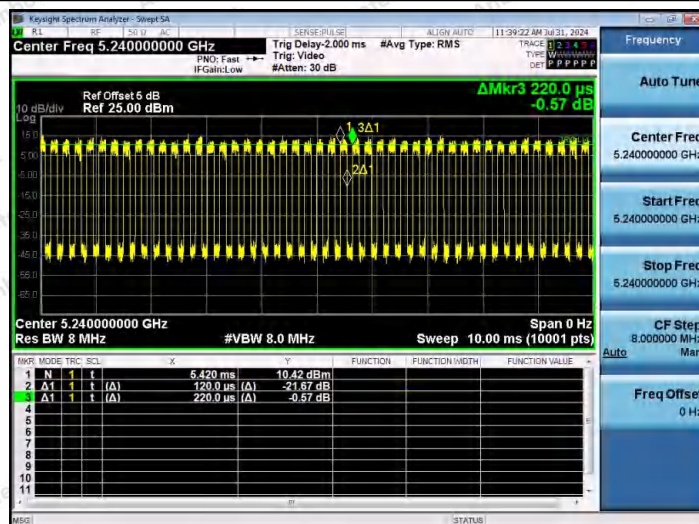
NTNV-11AX20MIMO-Ant1-5240
