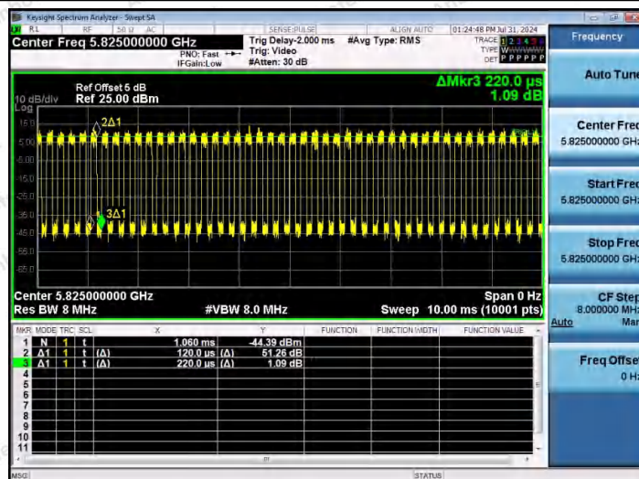
NTNV-11AX20MIMO-Ant1-5825
