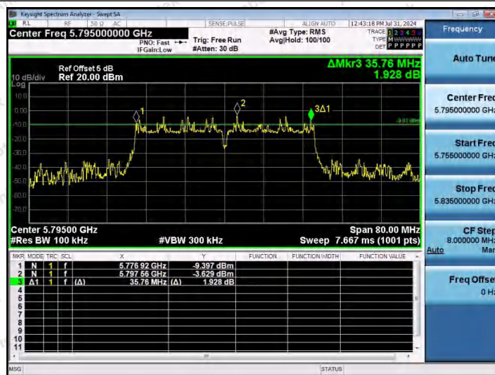
11N40MIMO-Ant1-5795-PASS
