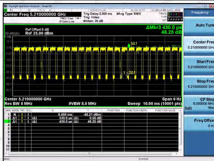
NTNV-11AC80MIMO-Ant1-5210
