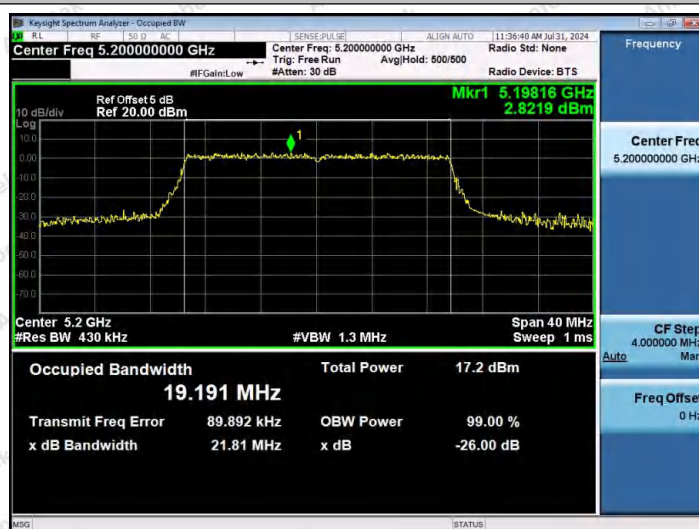
11AX20MIMO-Ant1-5200
