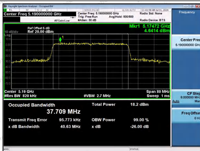
11AX40MIMO-Ant1-5190
