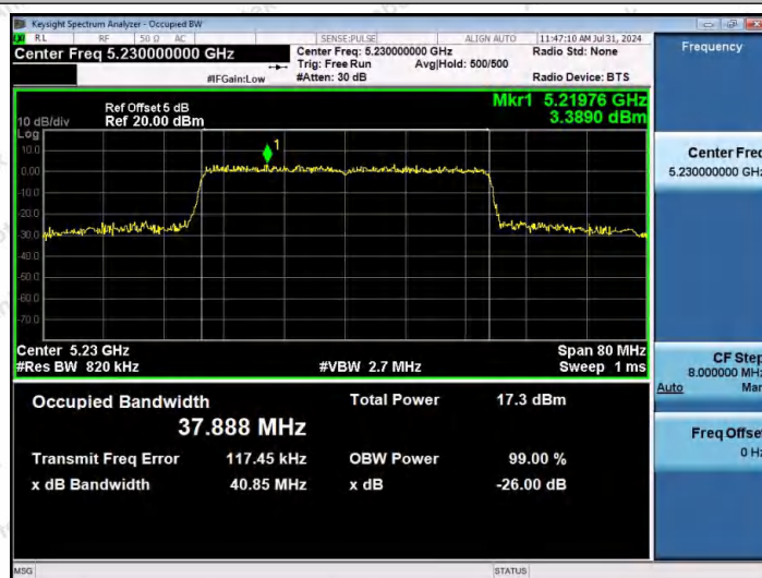
11AX40MIMO-Ant2-5230
