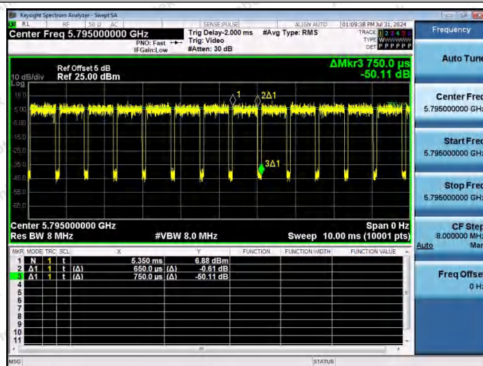
NTNV-11AC40MIMO-Ant1-5795
