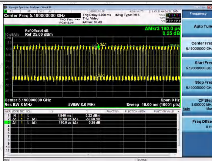
NTNV-11AX40MIMO-Ant1-5190
