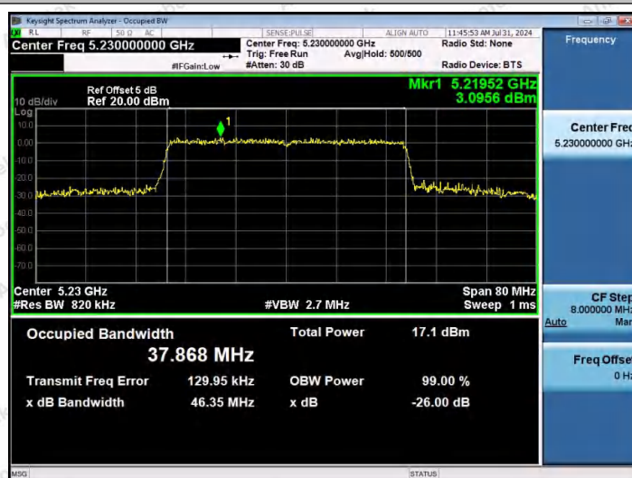
11AX40MIMO-Ant1-5230
