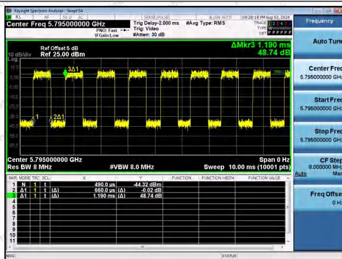
NTNV-11AX40MIMO-Ant1-5795
