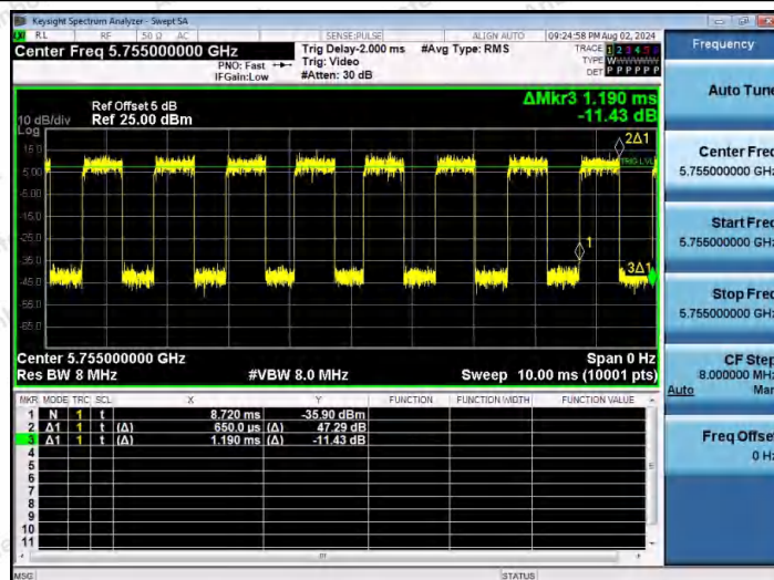
NTNV-11AX40MIMO-Ant1-5755
