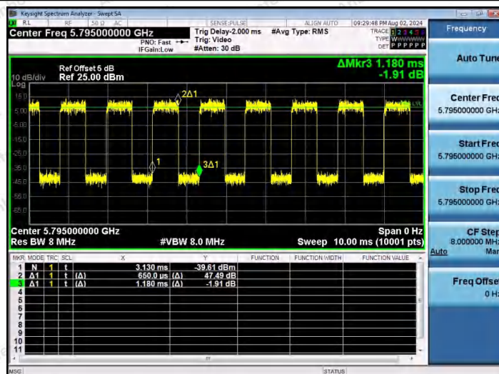
NTNV-11AX40MIMO-Ant2-5795
