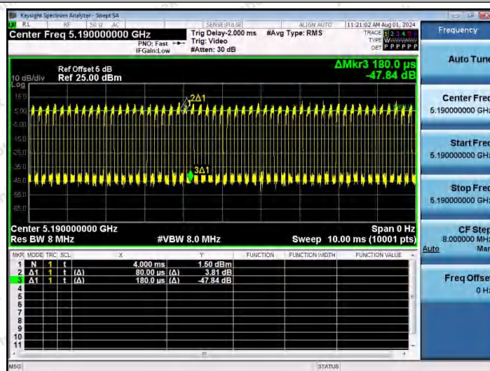
NTNV-11AX40MIMO-Ant1-5190
