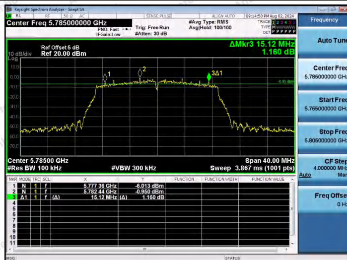
11AX20MIMO-Ant1-5785-PASS
