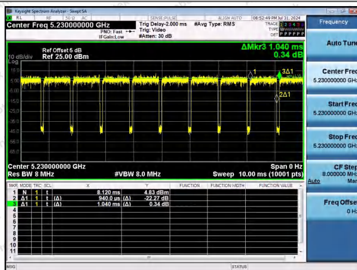
NTNV-11N40MIMO-Ant1-5230
