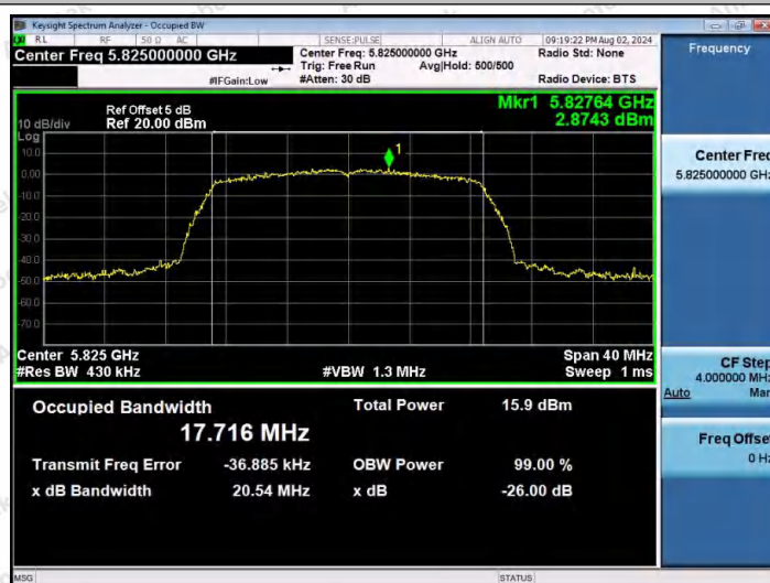
11AX20MIMO-Ant2-5825
