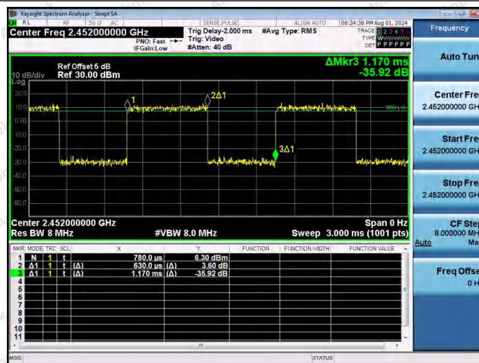
NTNV-11AX40MIMO-Ant1-2452
