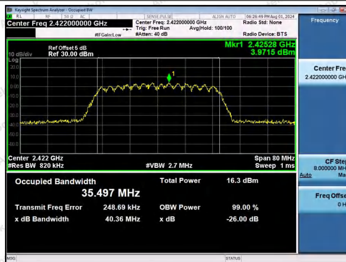
11AX40MIMO-Ant2-2422
