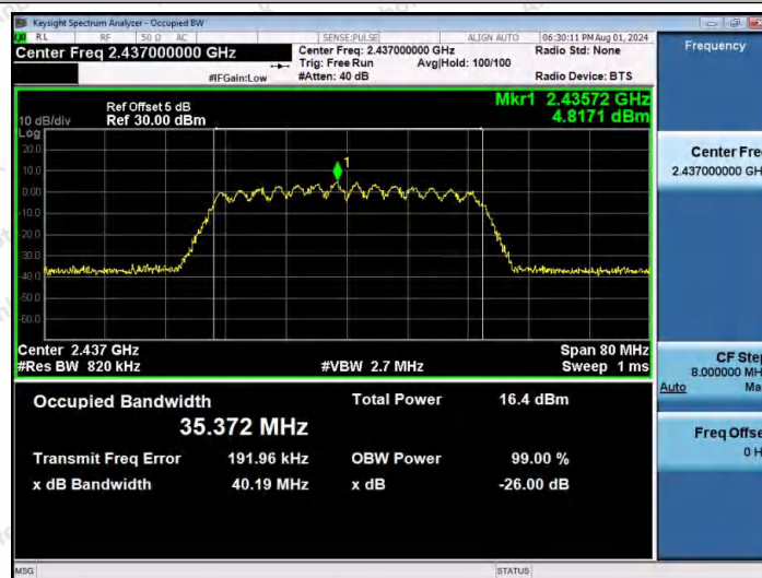
11AX40MIMO-Ant1-2437
