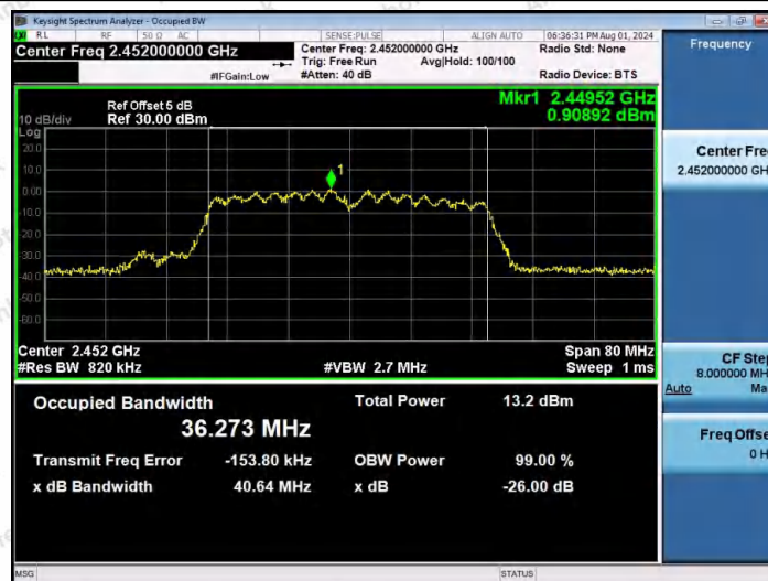
11AX40MIMO-Ant2-2452
