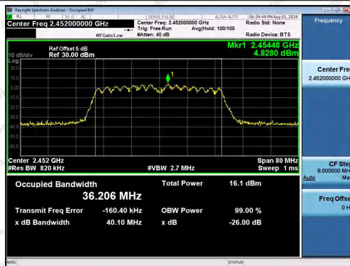
11AX40MIMO-Ant1-2452
