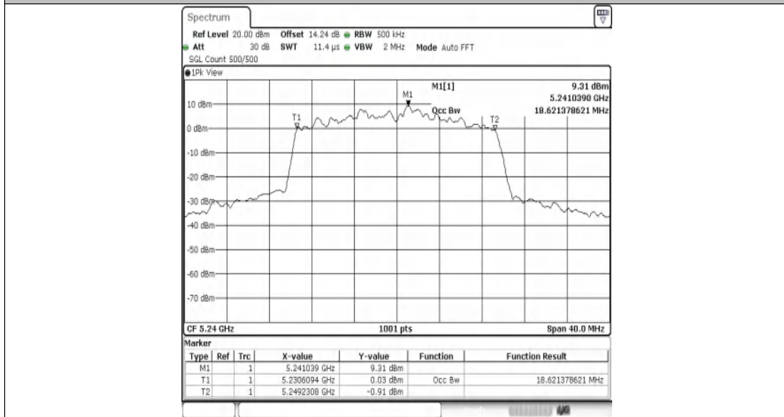
11AX20MIMO-Ant1-5240
