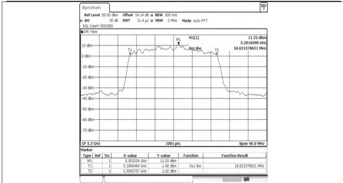
11AX20MIMO-Ant1-5200
