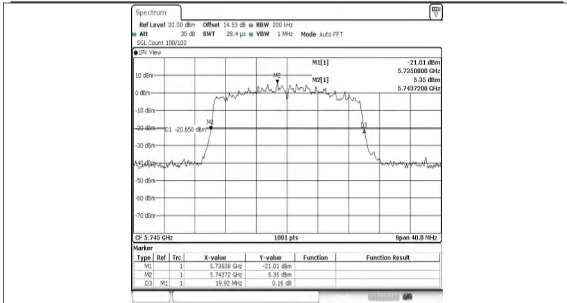
11AX20MIMO-Ant1-5745
