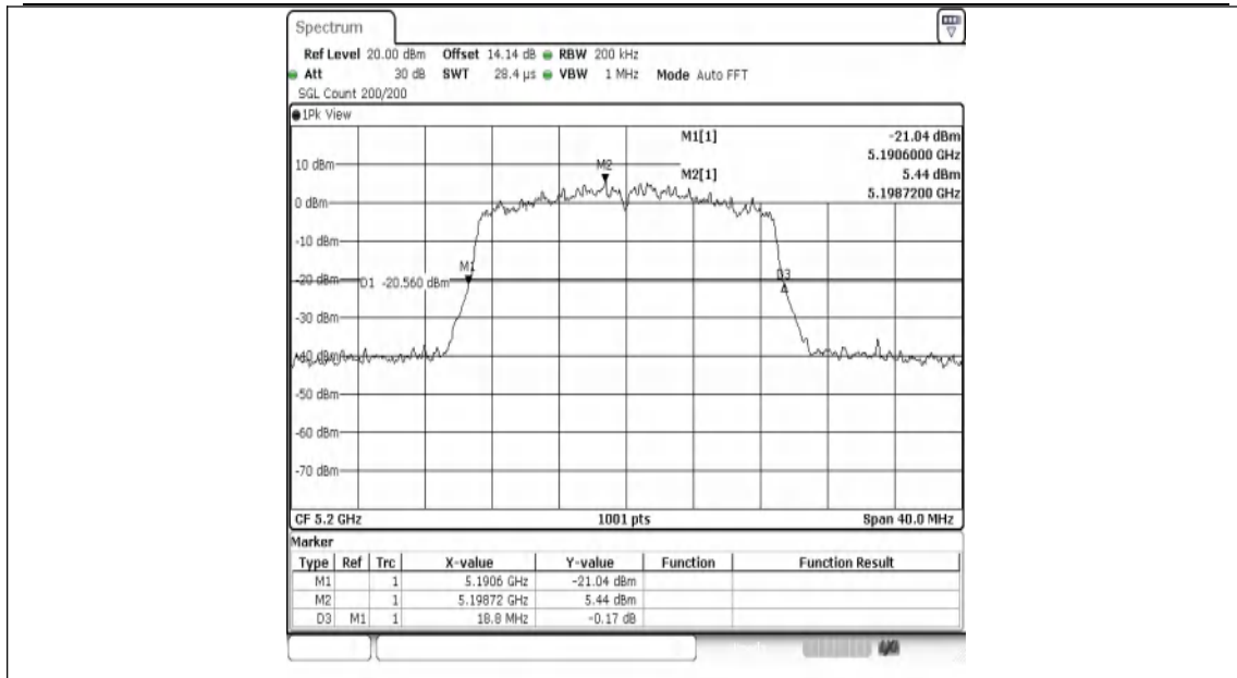
11N20MIMO-Ant1-5200
