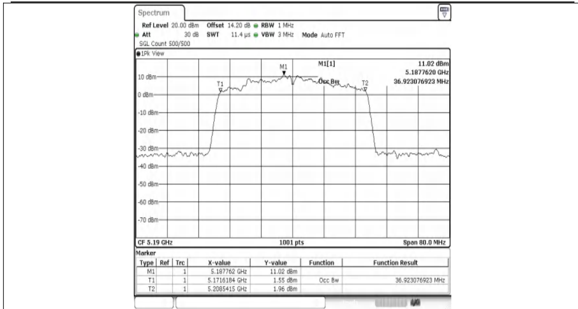
11AX40MIMO-Ant1-5190
