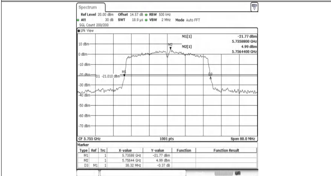
11AC40MIMO-Ant1-5755
