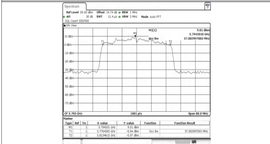
11AX40MIMO-Ant1-5795
