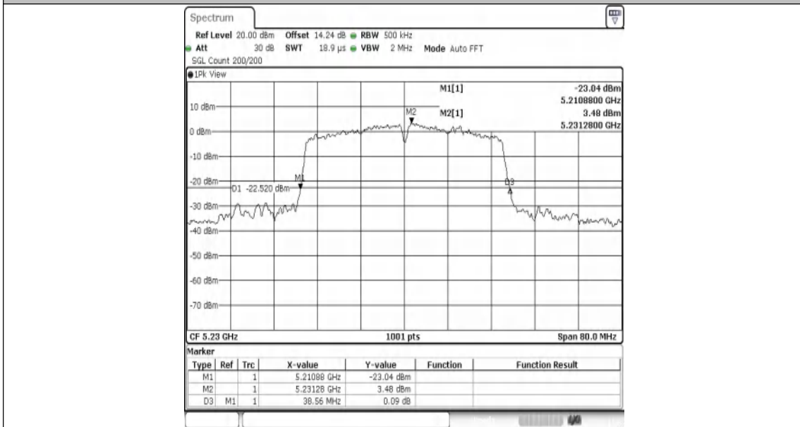
11AC40MIMO-Ant1-5230
