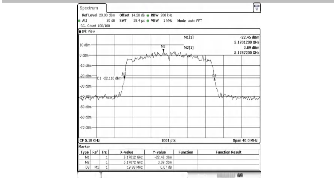
11AX20MIMO-Ant1-5180
