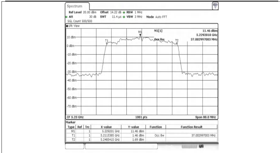
11AX40MIMO-Ant1-5230
