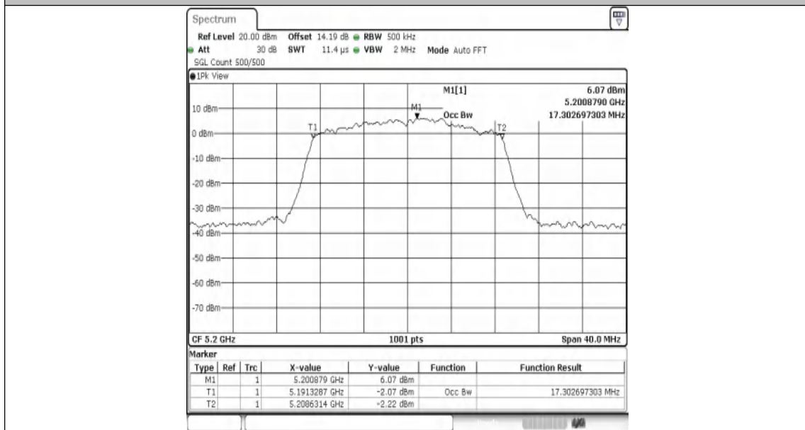
11AC20MIMO-Ant1-5200
