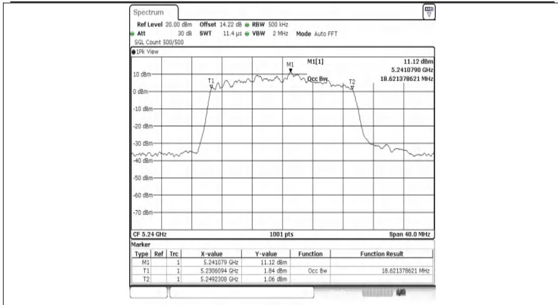
11AX20MIMO-Ant1-5240
