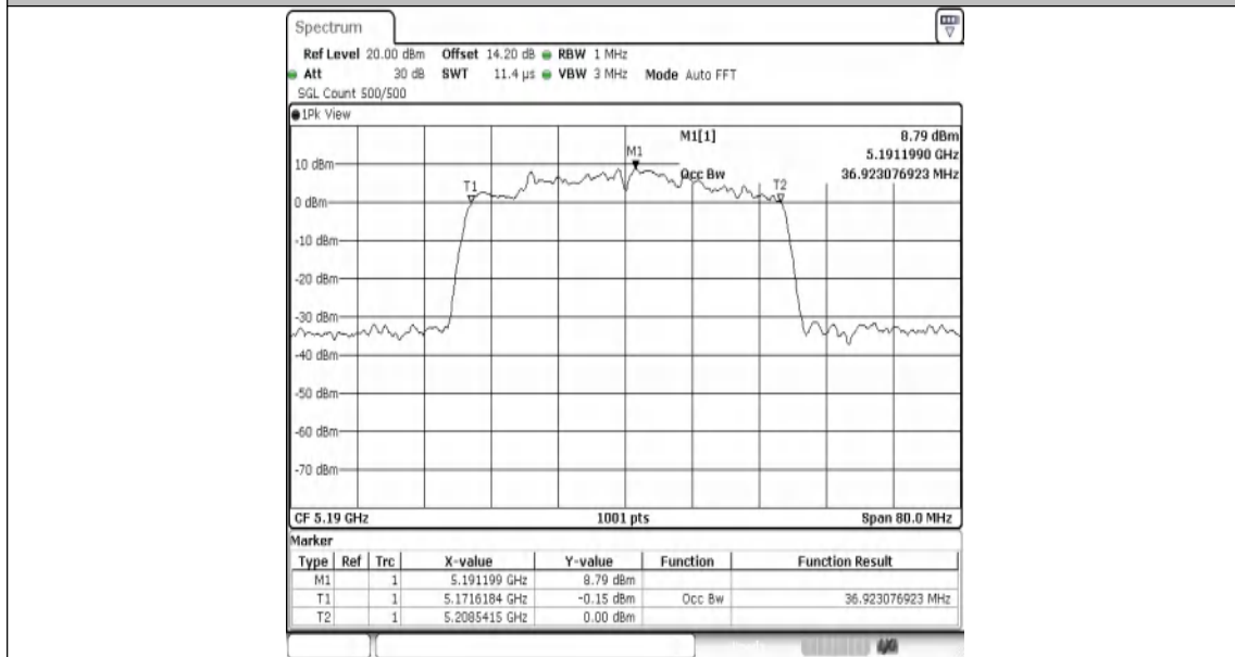
11AX40MIMO-Ant1-5190
