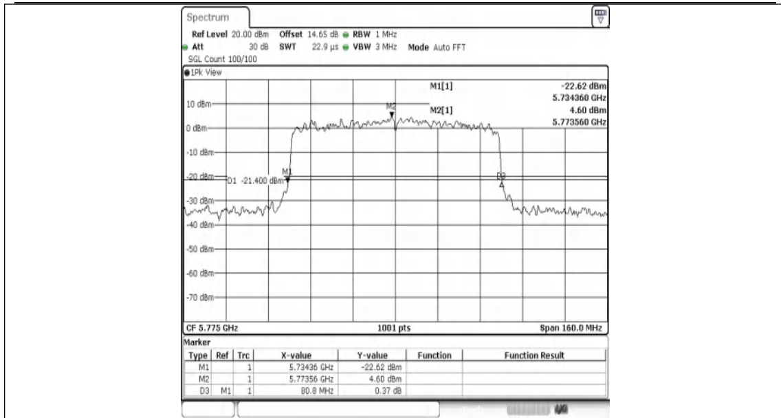
11AX80MIMO-Ant1-5775
