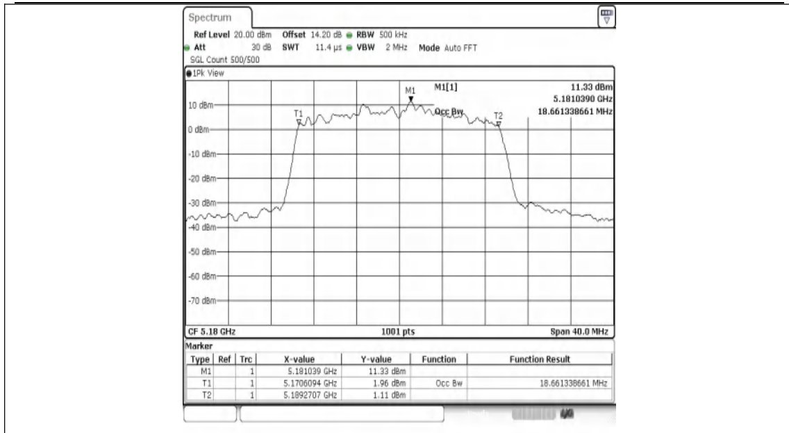
11AX20MIMO-Ant1-5180
