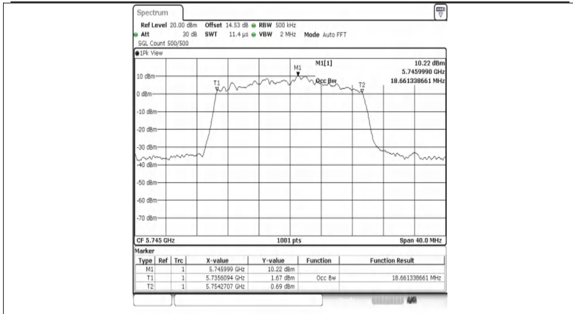
11AX20MIMO-Ant1-5745
