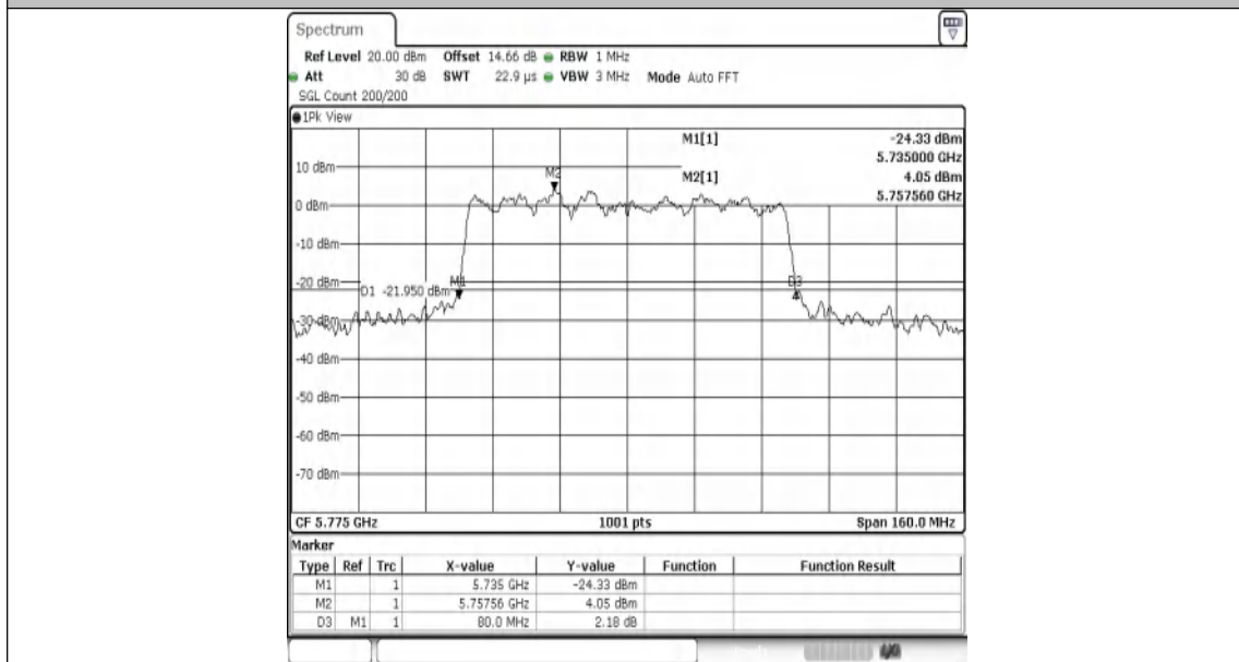
11AC80MIMO-Ant1-5775
