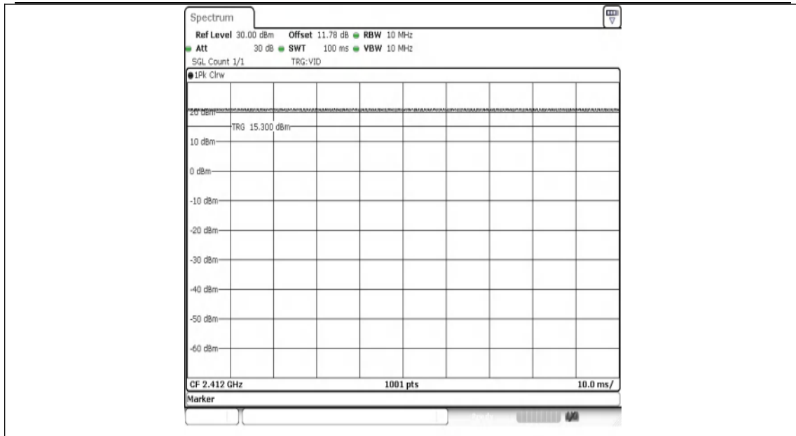
NTNV-11AX20MIMO-Ant1-2412
