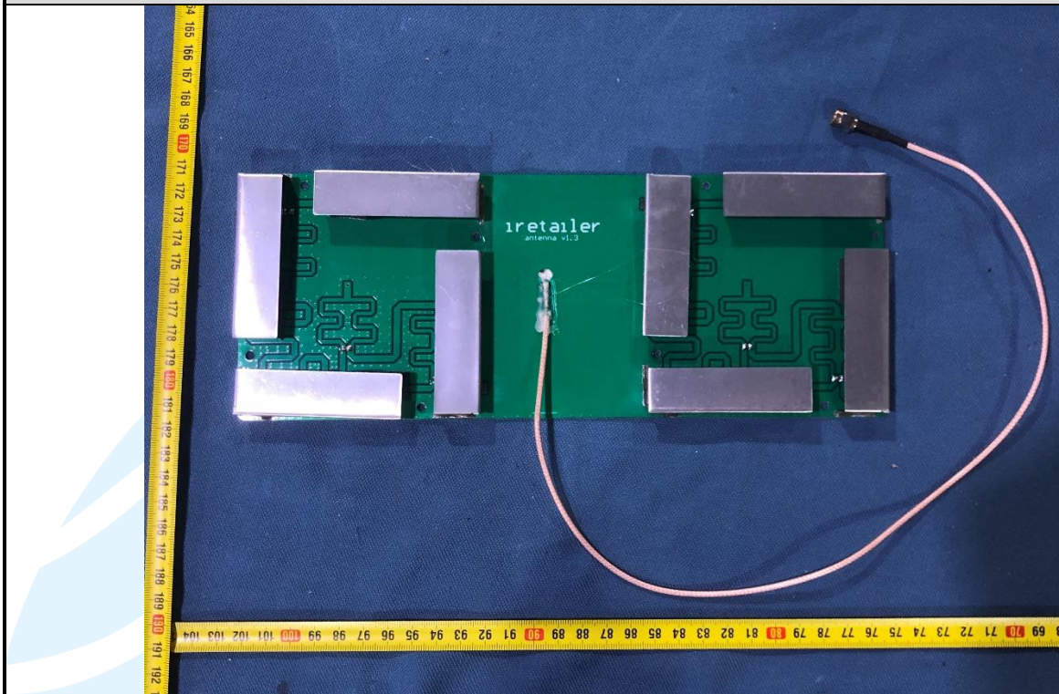
EUT Photo (Antenna)
