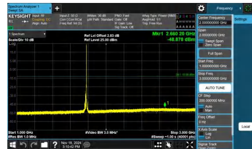
Band66-20MHz-QPSK-132572-1RB#99-1000~3000-PASS
