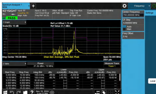
NTNV-Band14-10MHz-QPSK-23330-1RB#49--25.00--10.00-PASS
