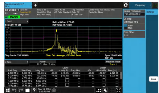
NTNV-Band14-5MHz-QPSK-23305-1RB#0--5.00--2.50-PASS
