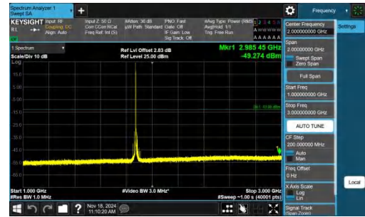
Band2-20MHz-QPSK-18900-1RB#0-1000~3000-PASS
