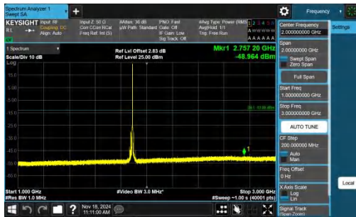
Band2-20MHz-QPSK-18900-1RB#99-1000~3000-PASS
