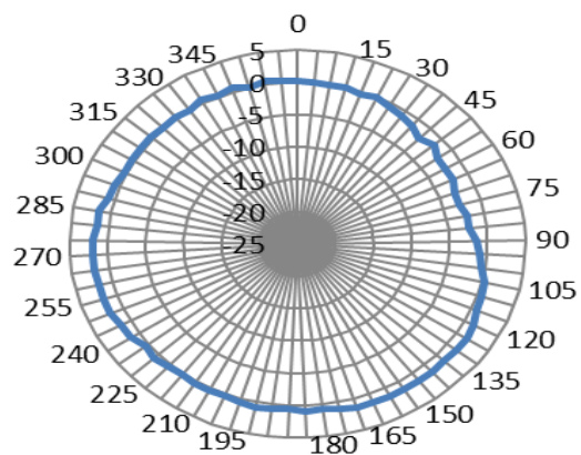
XY-5500MHz
