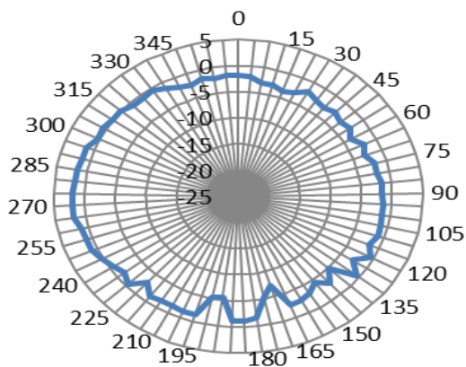
YZ-5500MHz
