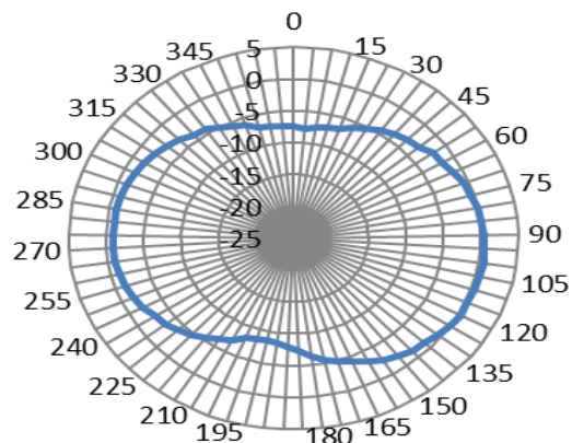
XY-2450MHz
