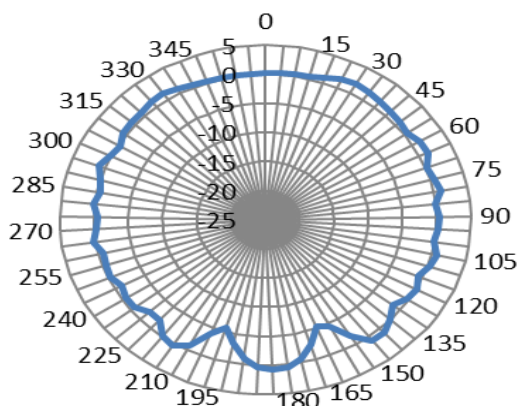
YZ-2450MHz
