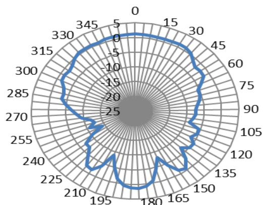
XZ-2450MHz
