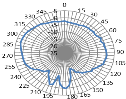
XZ-5500MHz
