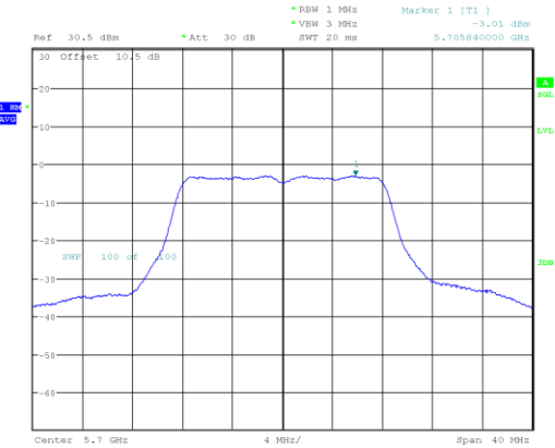
802.11a mode, 5700MHz
