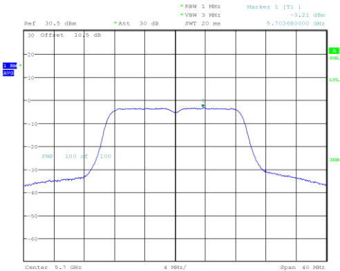
802.11n-HT20 mode, 5700MHz
