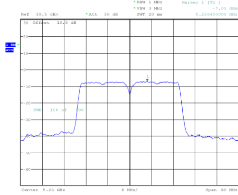
802.11n-HT40 mode, 5230MHz
