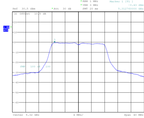
802.11a mode, 5320MHz
