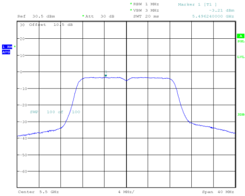
802.11n-HT20 mode, 5500MHz
