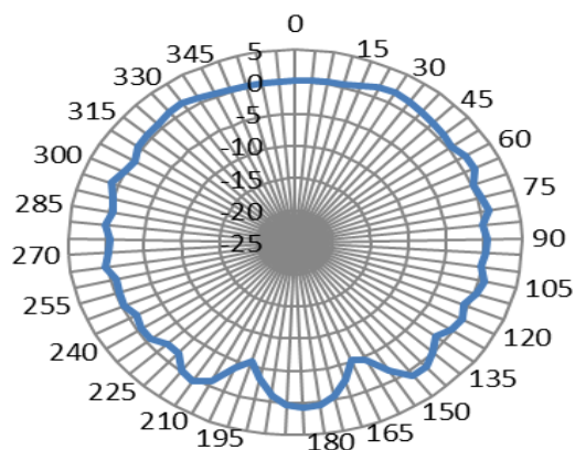
YZ-2450MHz
