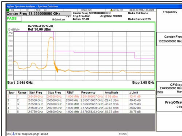
B41(2535-2655) / 10MHz / High CH / QPSK / 1 RB
