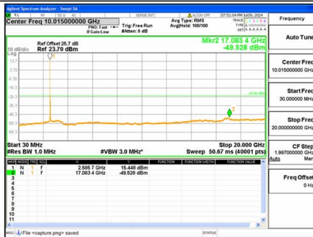
B41(2535-2655)-30M-20G / 20MHz / Mid CH / QPSK
