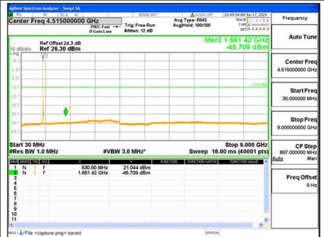
B19 / 10MHz / Low CH / QPSK
