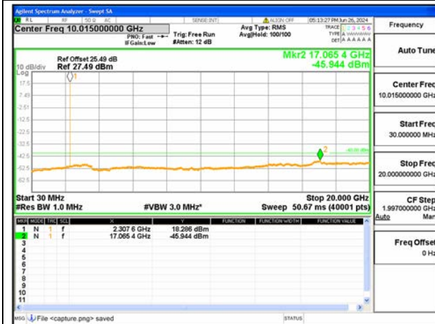
B40-1-30M-20G / 5MHz / Mid CH / QPSK
