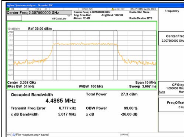
B40-1 / 5MHz / 64QAM / Low CH
