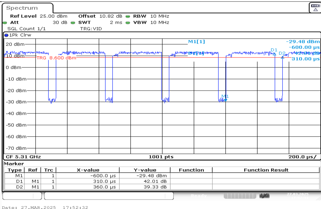
NTNV-11AX40MIMO-Ant1-5310
