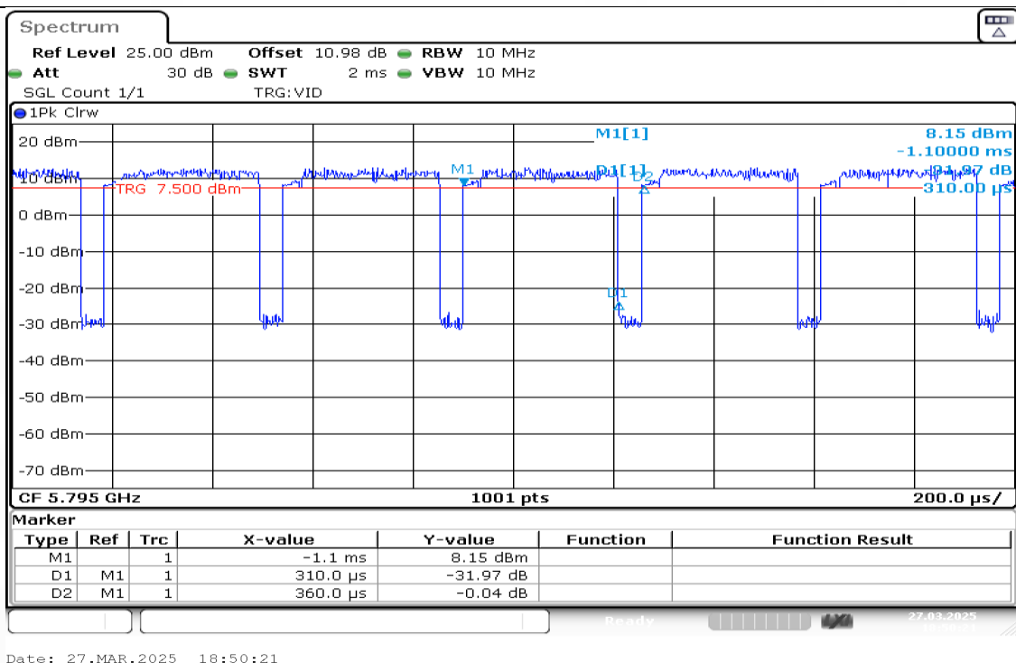
NTNV-11AX40MIMO-Ant1-5795
