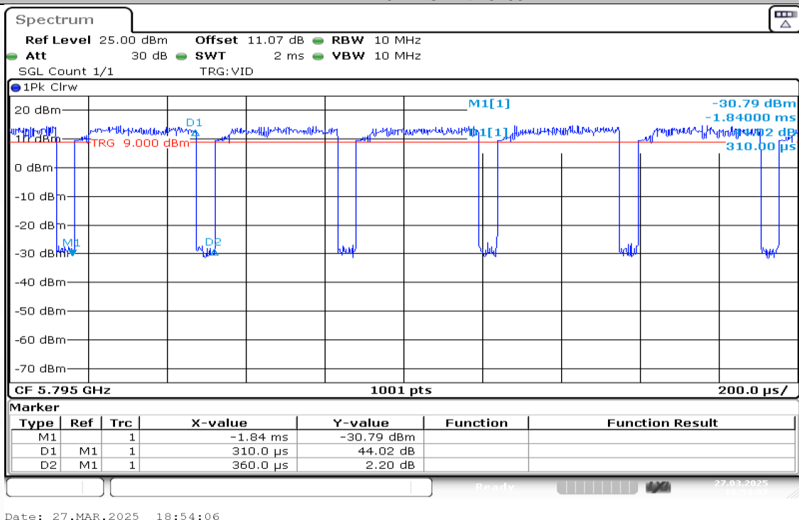
NTNV-11AX40MIMO-Ant2-5795
