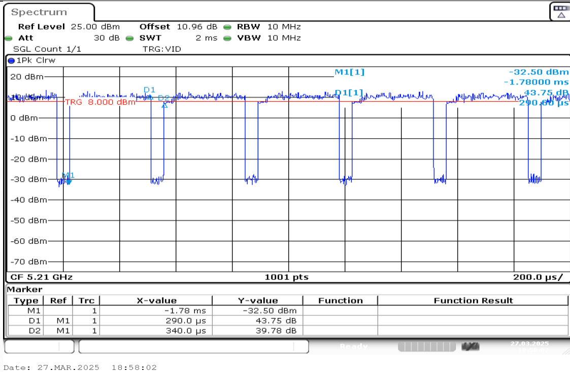
NTNV-11AX80MIMO-Ant1-5210
