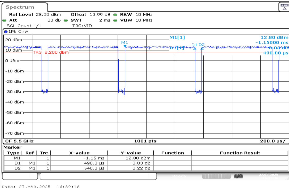
NTNV-11AX20MIMO-Ant1-5500
