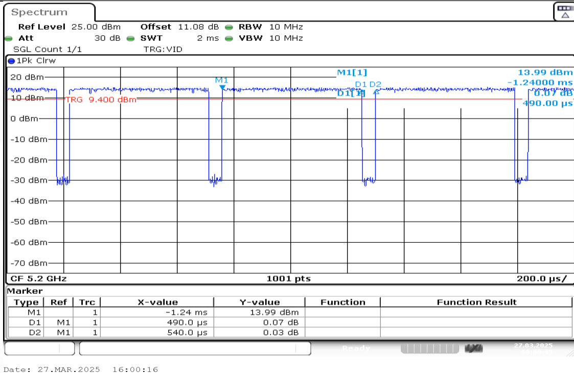
NTNV-11AX20MIMO-Ant2-5200
