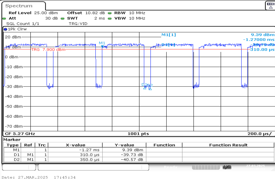
NTNV-11AX40MIMO-Ant1-5270
