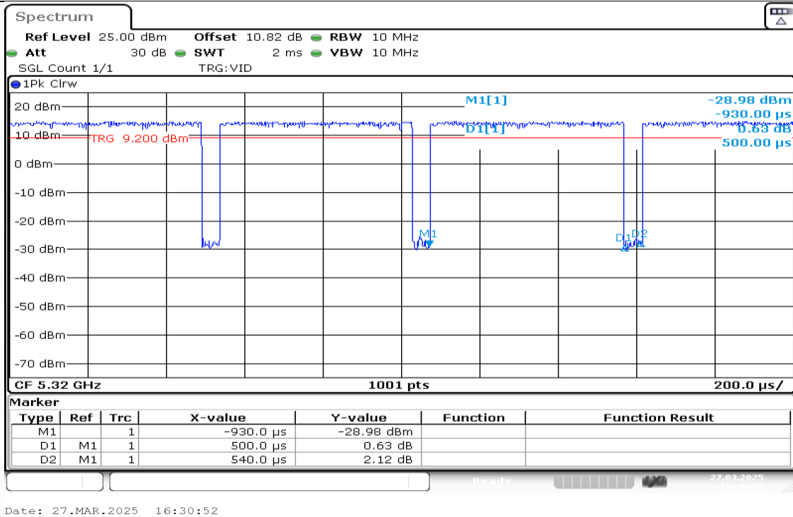
NTNV-11AX20MIMO-Ant1-5320
