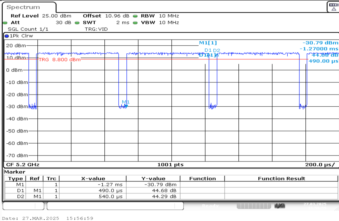
NTNV-11AX20MIMO-Ant1-5200
