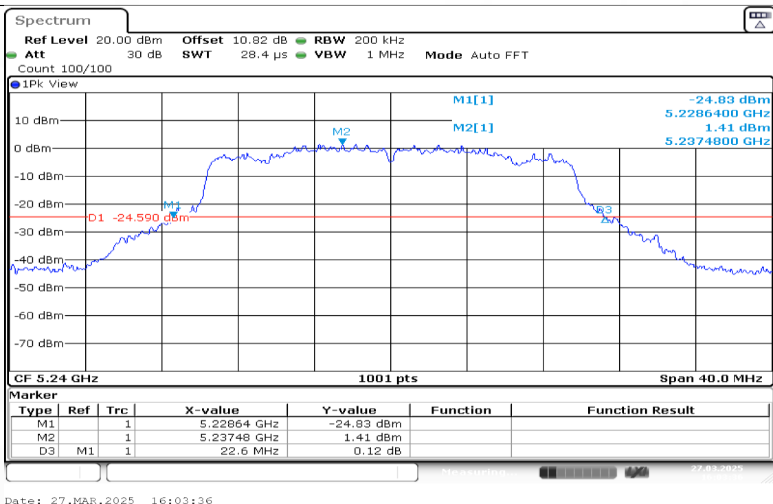
11AX20MIMO-Ant1-5240
