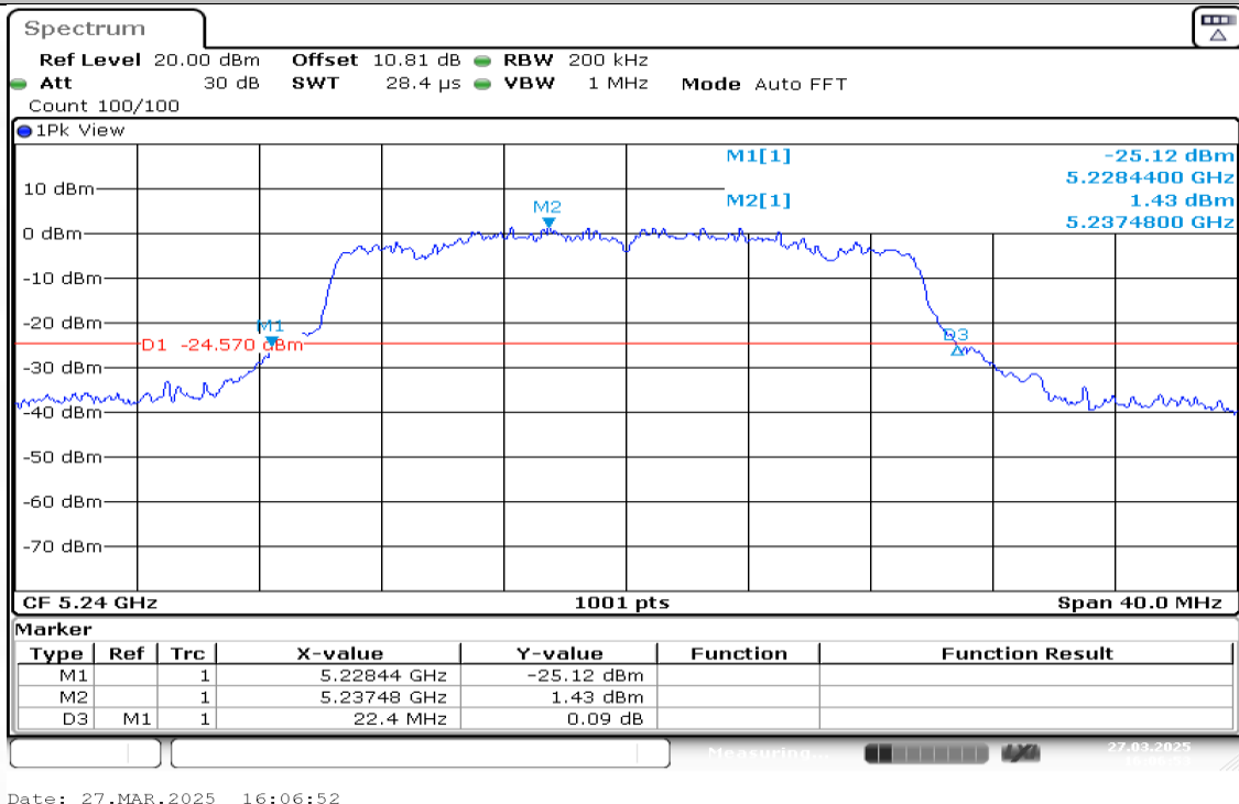
11AX20MIMO-Ant2-5240
