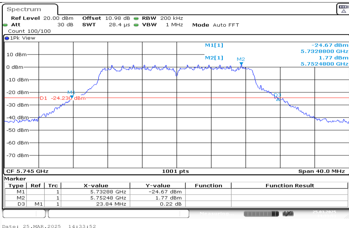
11N20MIMO-Ant1-5745
