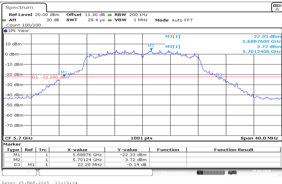
11A-Ant1-5700
