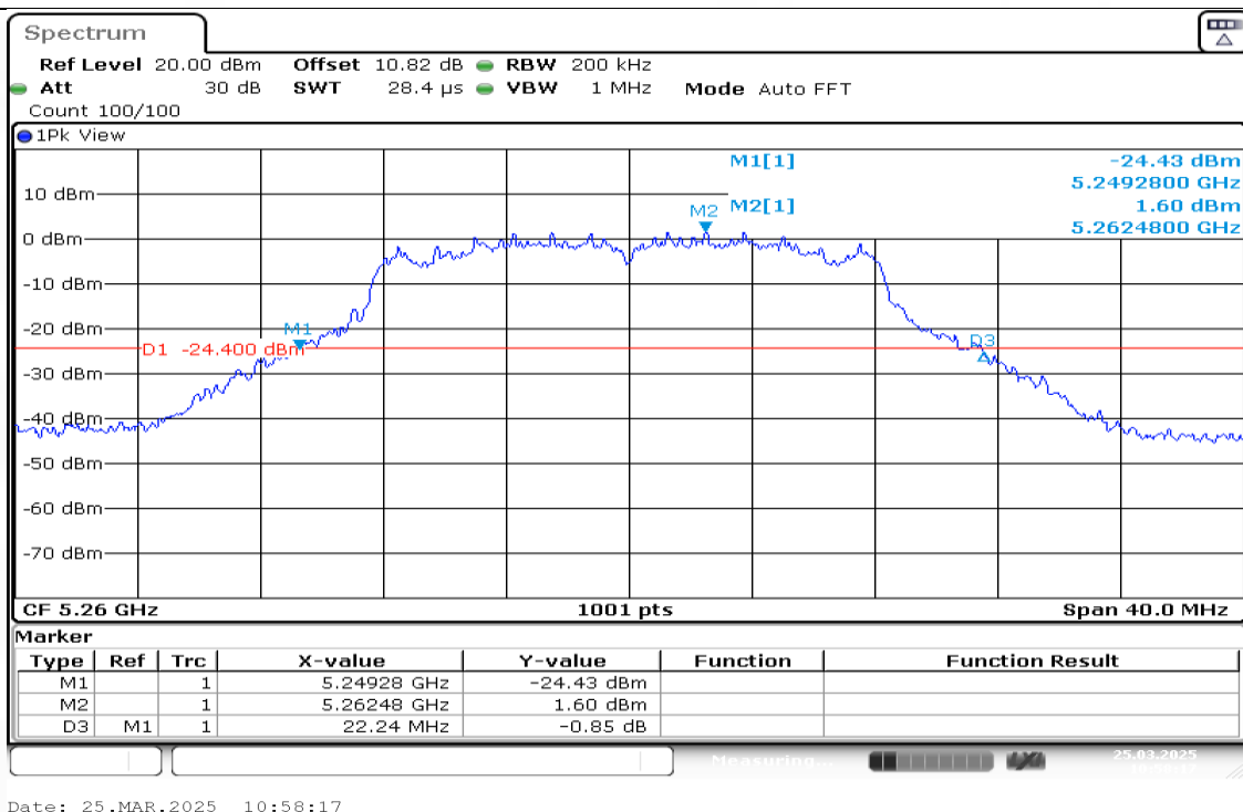
11A-Ant1-5260
