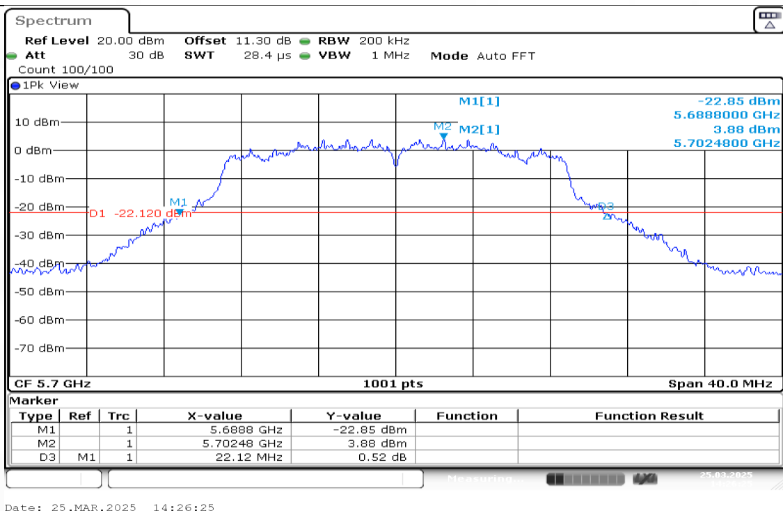
11N20MIMO-Ant1-5700
