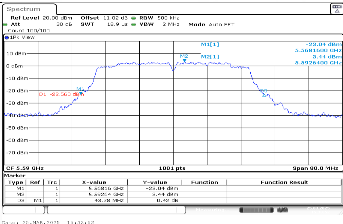
11N40MIMO-Ant1-5590
