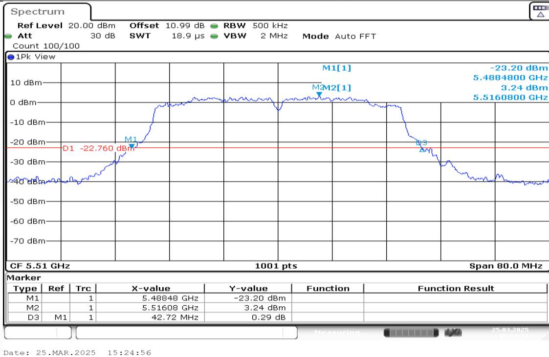
11N40MIMO-Ant1-5510
