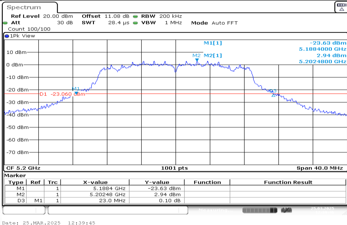
11N20MIMO-Ant2-5200
