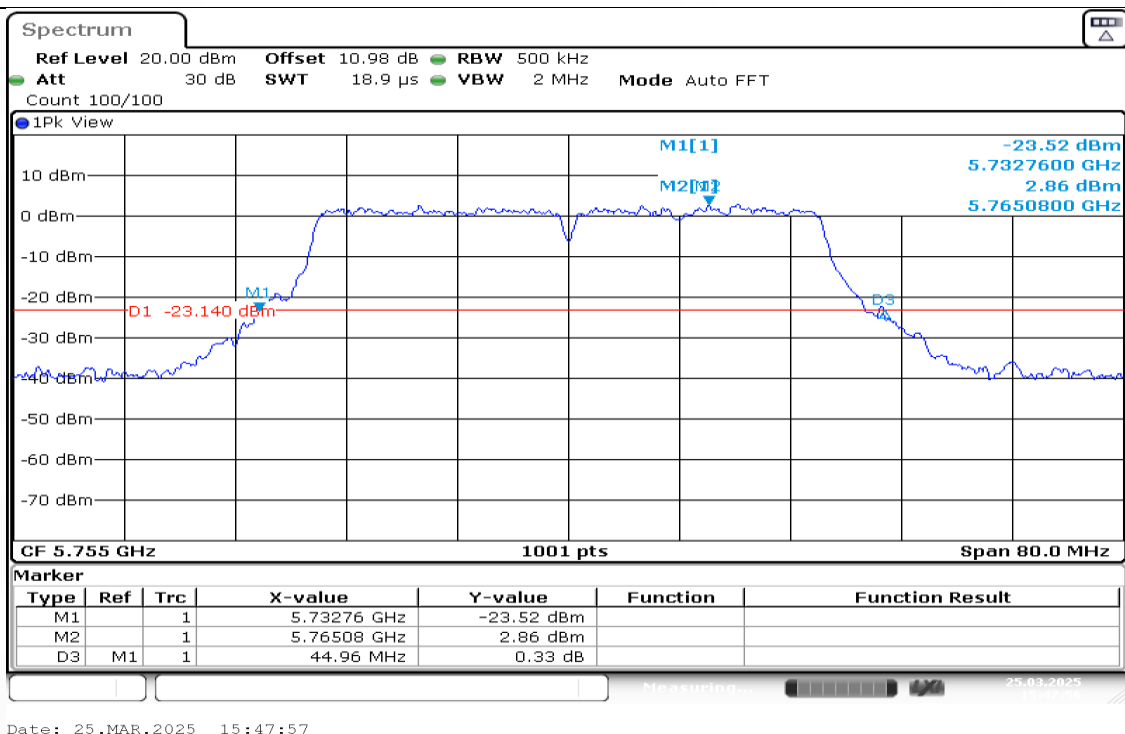
11N40MIMO-Ant1-5755
