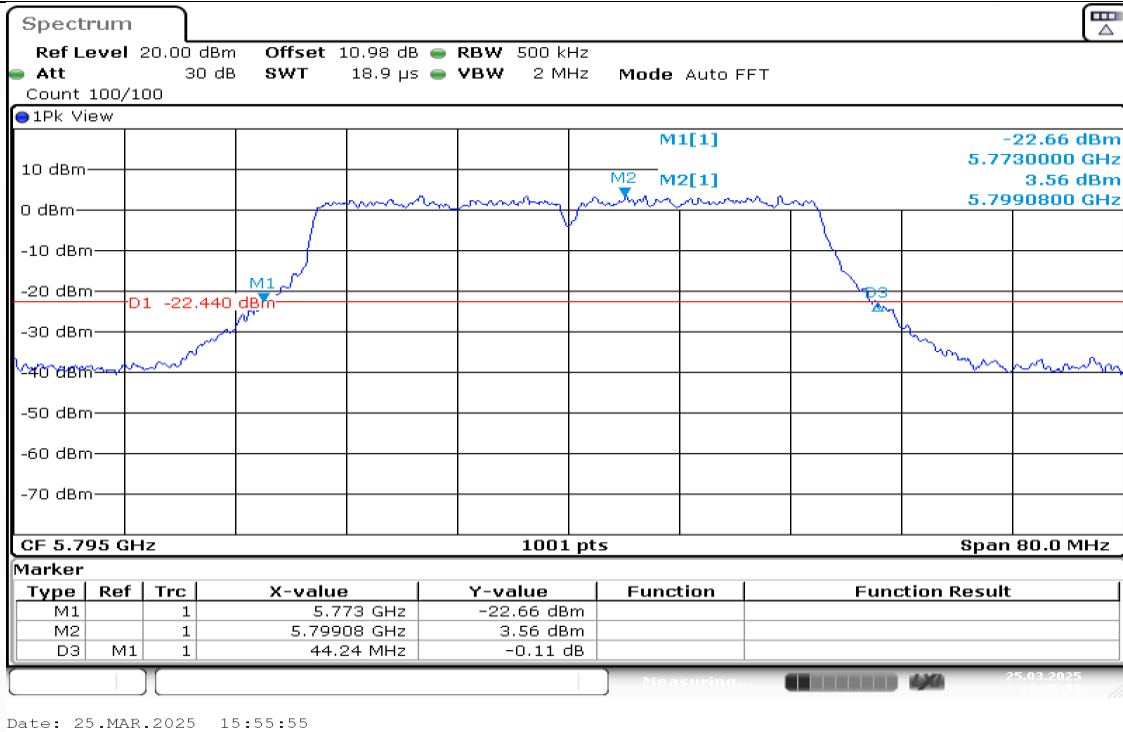
11N40MIMO-Ant1-5795
