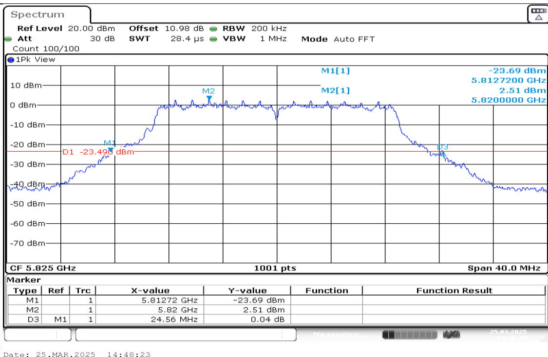
11N20MIMO-Ant1-5825
