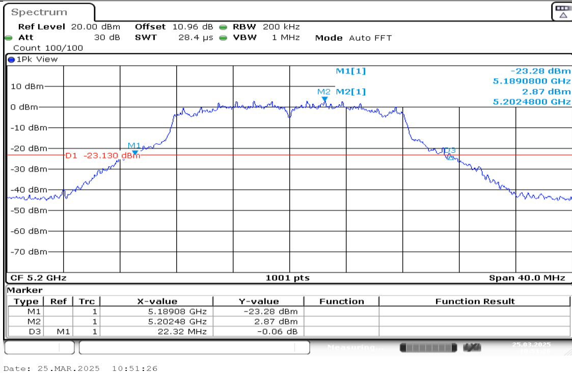
11A-Ant1-5200
