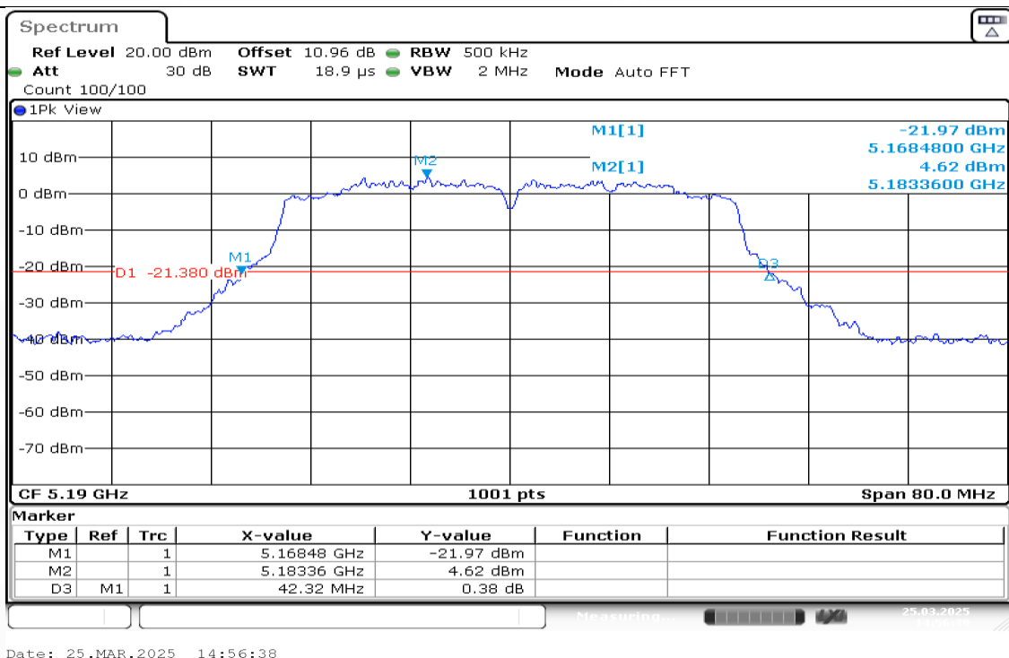
11N40MIMO-Ant1-5190
