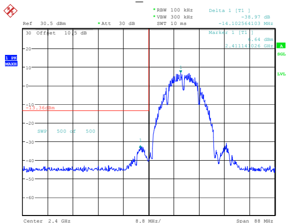
802.11b 2412MHz
