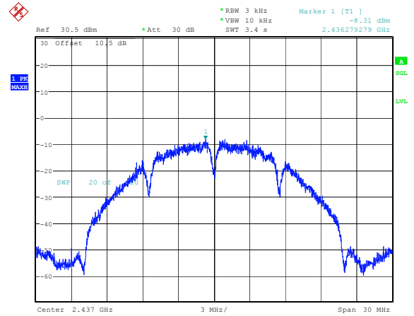
802.11b_2437MHz -8.31dBm/3kHz
