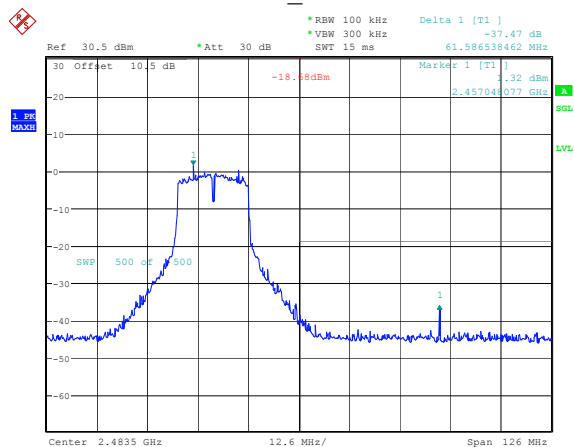
802.11n20 2462MHz
