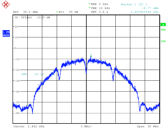
802.11b_2462MHz -8.77dBm/3kHz
