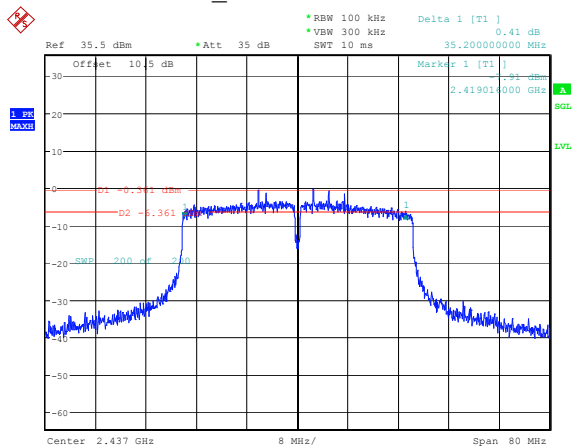
802.11n40_2437MHz 35.200MHz
