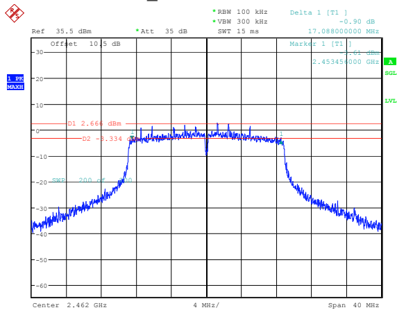
802.11n20_2462MHz 17.088MHz
