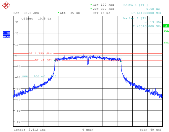
802.11n20_2412MHz 17.664MHz
