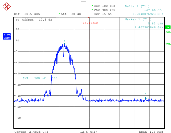
802.11b 2462MHz
