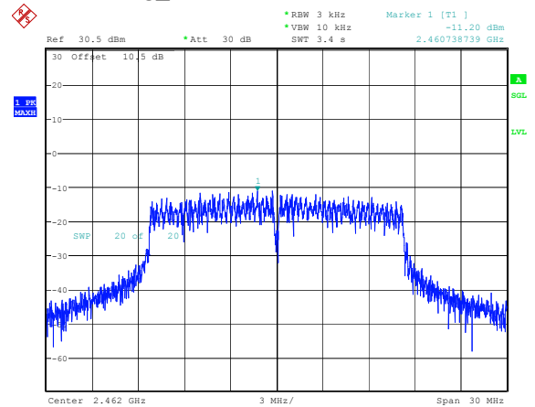
802.11g_2462MHz -11.20dBm/3kHz
