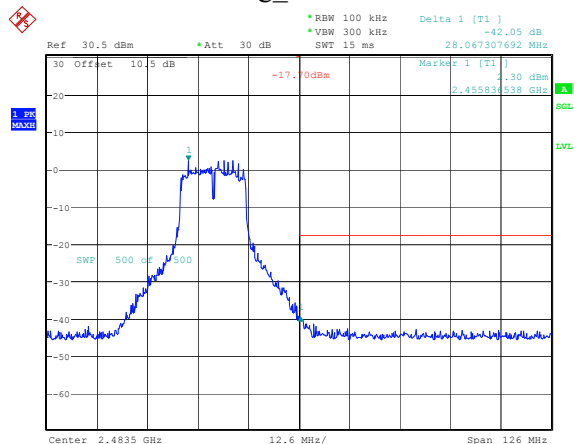
802.11g 2462MHz
