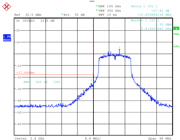
802.11n20 2412MHz
