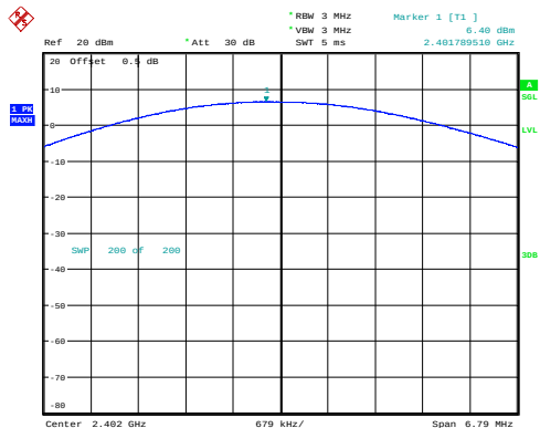
\pi/4 -DQPSK_Low 6.40dBm
