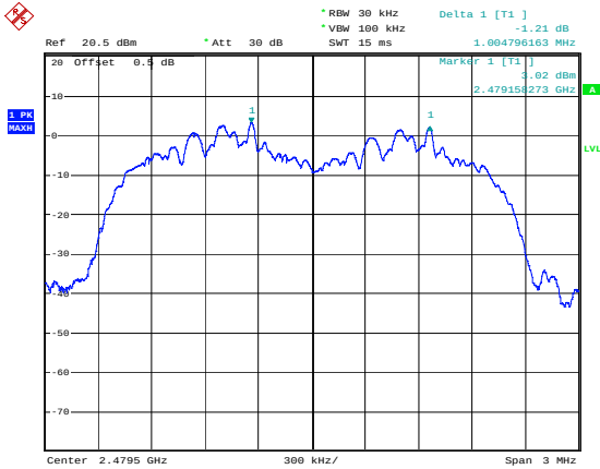
\pi/4 -DQPSK_High 1.005MHz
