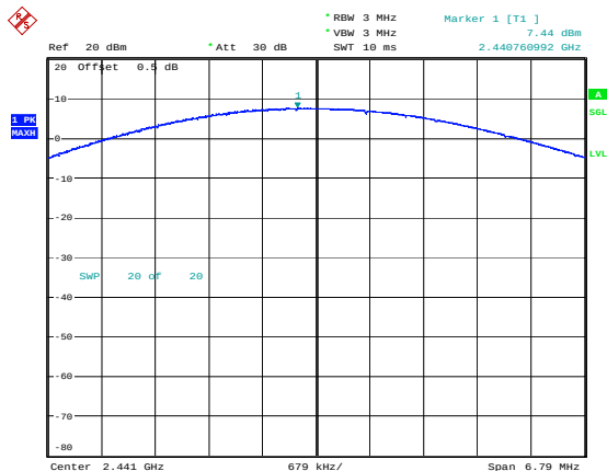
\pi/4 -DQPSK_Middle 7.44dBm
