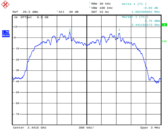
\pi/4 -DQPSK_Middle 1.002MHz
