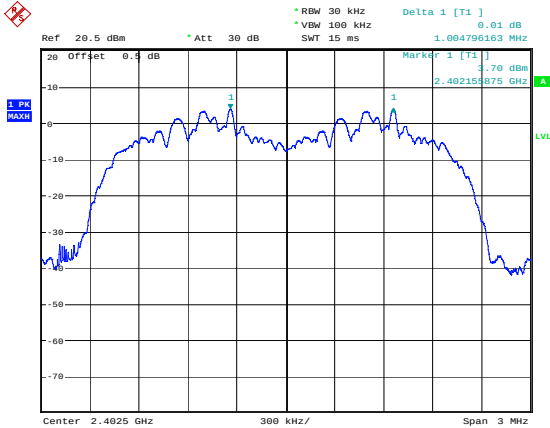
\pi/4 -DQPSK_Low 1.005MHz
