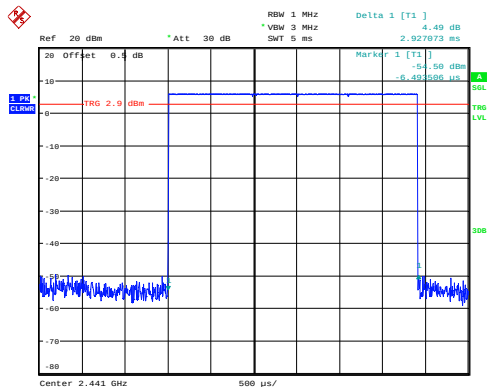
GFSK_Hopping_DH5 2.927ms
