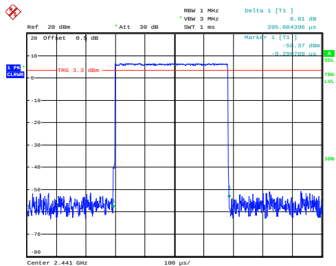
GFSK_Hopping_DH1 0.396ms
