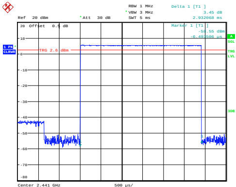
GFSK_Hopping_DH5 2.932ms
