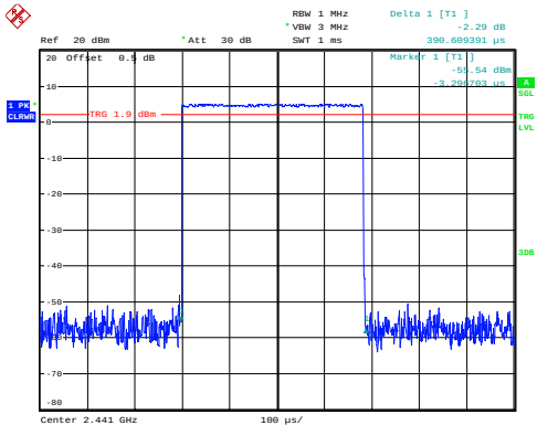
GFSK_Hopping_DH1 0.391ms
