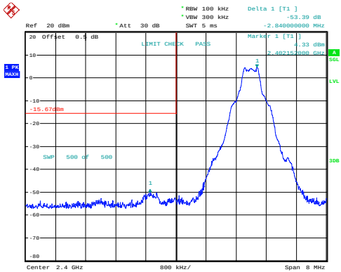
GFSK_Low 53.39dB
