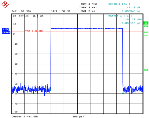
GFSK_Hopping_DH3 1.660ms
