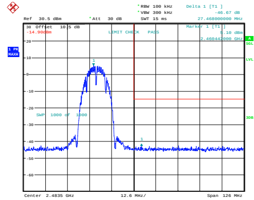
b_2462MHz_Chain 0 46.67dB
