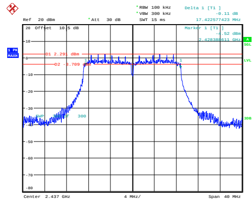
n20_2437MHz_Chain 0 17.423MHz
