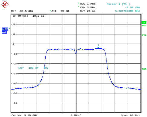
n40_5190MHz_Chain 0 -4.54dBm/MHz
