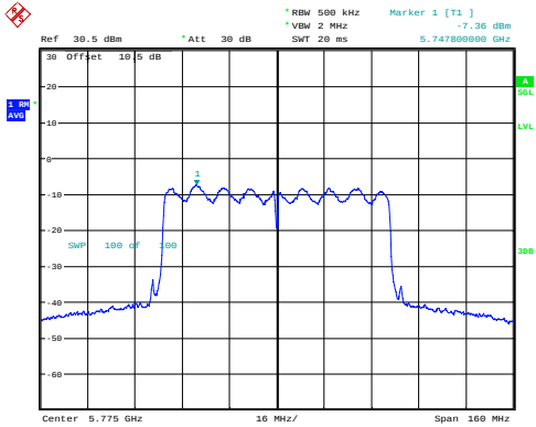
ac80_5775MHz_Chain 0 -7.36dBm/MHz
