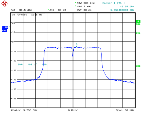
n40_5755MHz_Chain 0 -5.65dBm/MHz
