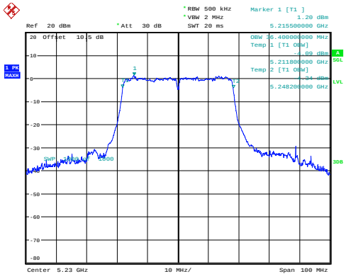
n40_5230MHz_Chain 0 36.400MHz
