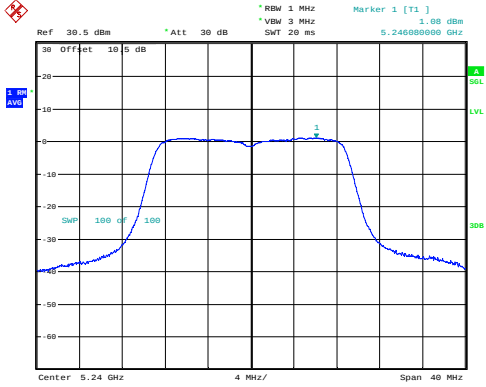
n20_5240MHz_Chain 0 1.08dBm/MHz
