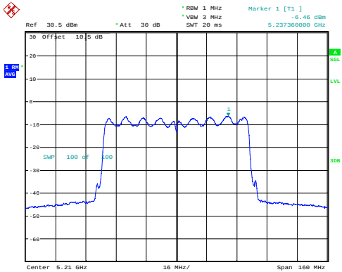
ac80_5210MHz_Chain 0 -6.46dBm/MHz
