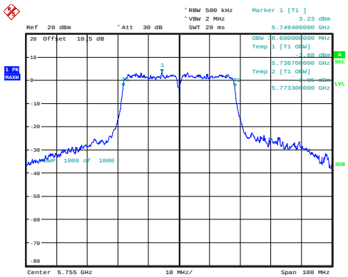
n40_5755MHz_Chain 0 36.600MHz
