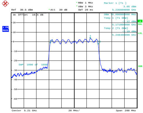
ac80_5210MHz_Chain 0 76.600MHz
