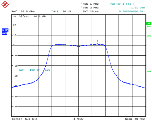
a_5200MHz_Chain 0 1.01dBm/MHz
