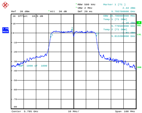
n40_5795MHz_Chain 0 36.700MHz
