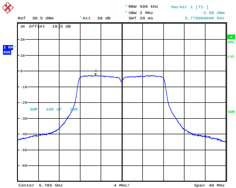
a_5785MHz_Chain 0 -2.90dBm/MHz
