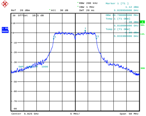
a_5825MHz_Chain 0 16.700MHz
