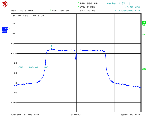
n40_5795MHz_Chain 0 -5.99dBm/MHz
