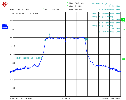
n40_5190MHz_Chain 0 36.400MHz
