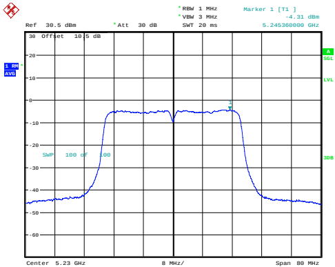
n40_5230MHz_Chain 0 -4.31dBm/MHz
