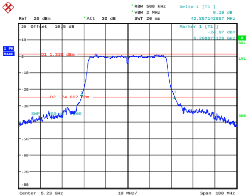
n40_5230MHz_Chain 0 42.857MHz
