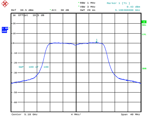
n20_5180MHz_Chain 0 0.43dBm/MHz
