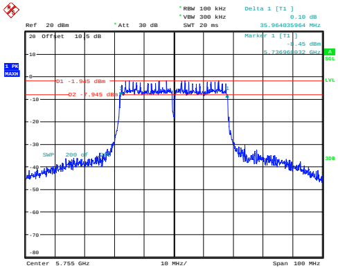
n40_5755MHz_Chain 0 35.964MHz
