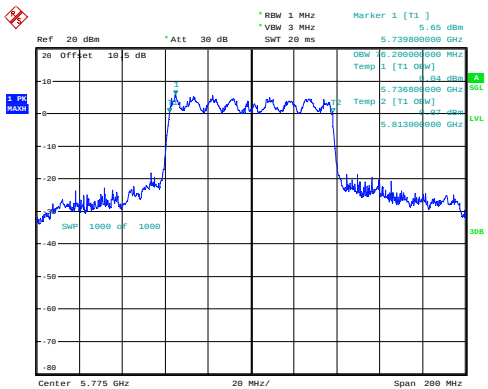
ac80_5775MHz_Chain 0 76.200MHz
