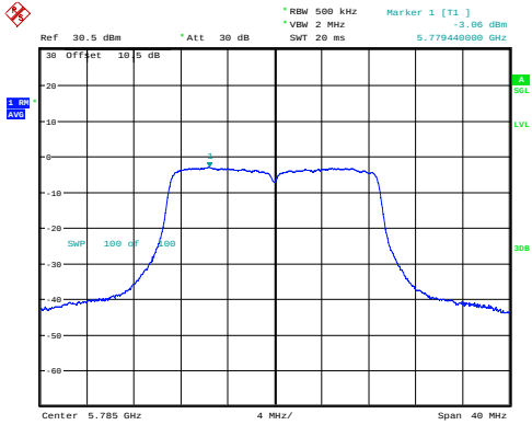
n20_5785MHz_Chain 0 -3.06dBm/MHz
