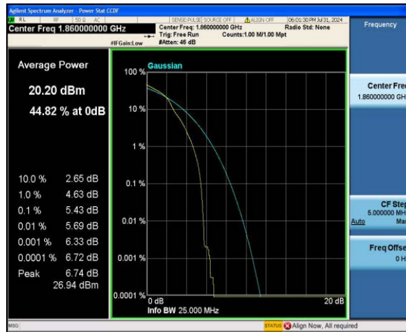
Band2-20MHz-16QAM-18700-100RB#0
