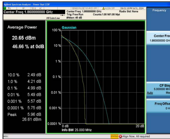
Band2-20MHz-QPSK-18700-100RB#0
