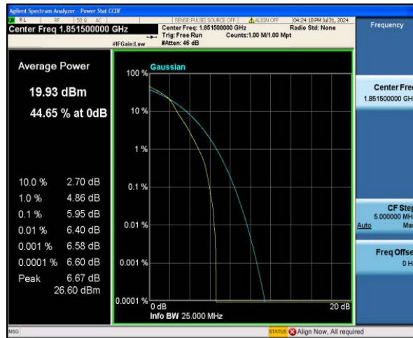
Band2-3MHz-16QAM-18615-15RB#0
