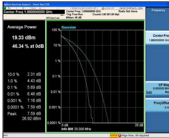
Band2-20MHz-QPSK-19100-1RB#0
