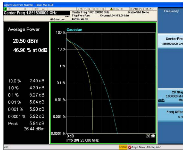
Band2-3MHz-QPSK-18615-15RB#0
