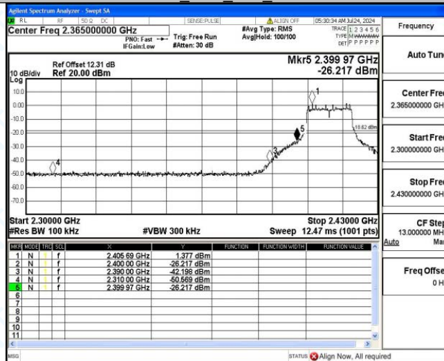
11G_Ant1_Low_2412
