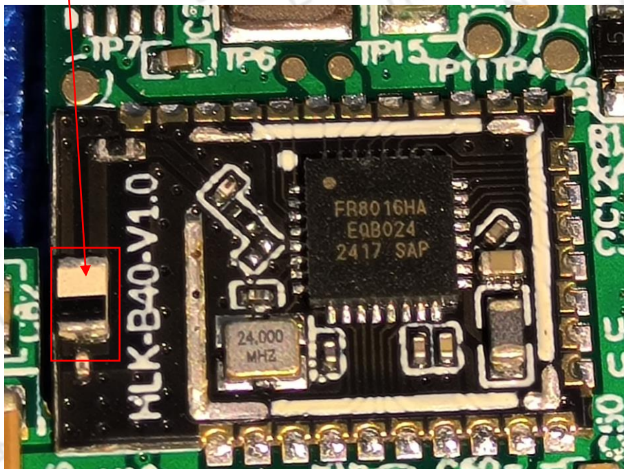
BLE Antenna
