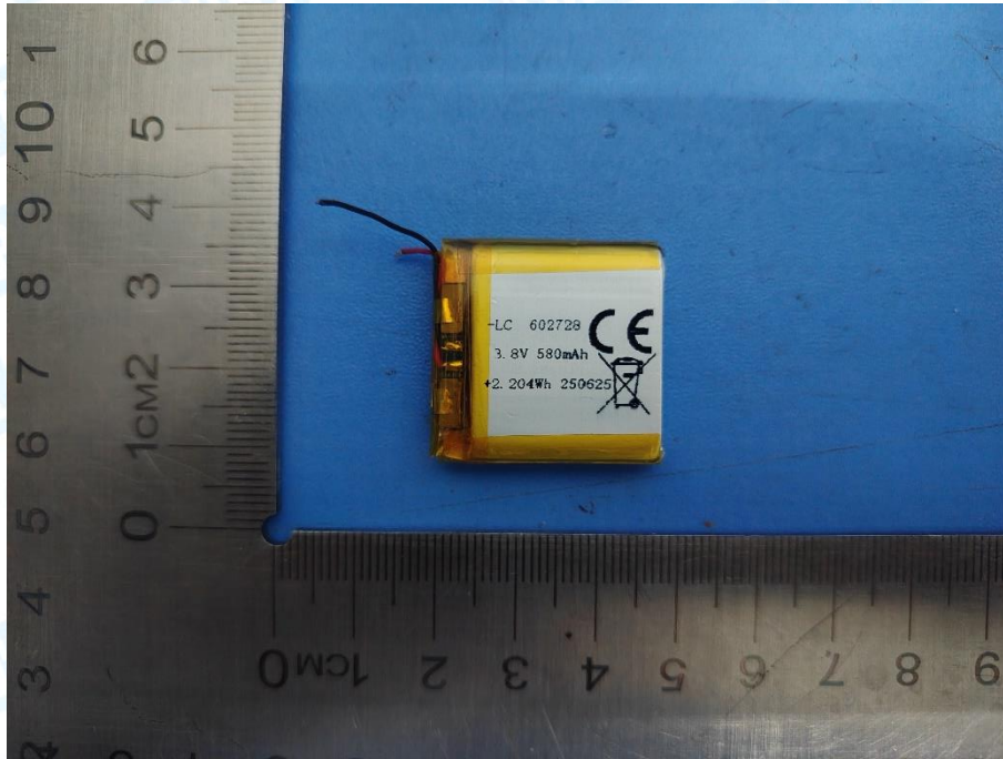
Photo 16 Battery parameters
