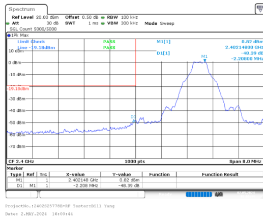
GFSK_Low_DH1
