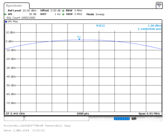
\pi/4 -DQPSK_Mid_2DH1
