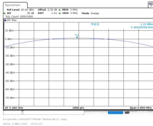
\pi/4 -DQPSK_Low_2DH1
