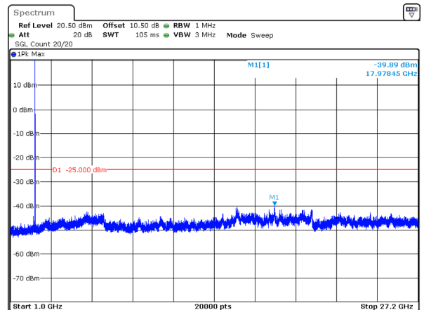
5MHz_Low_QPSK_25@0(1GHz~27.2GHz)
