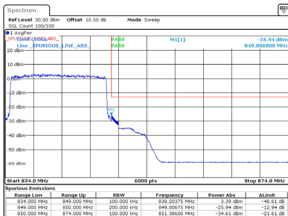
B26_2_15MHz_High_QPSK_75@0
