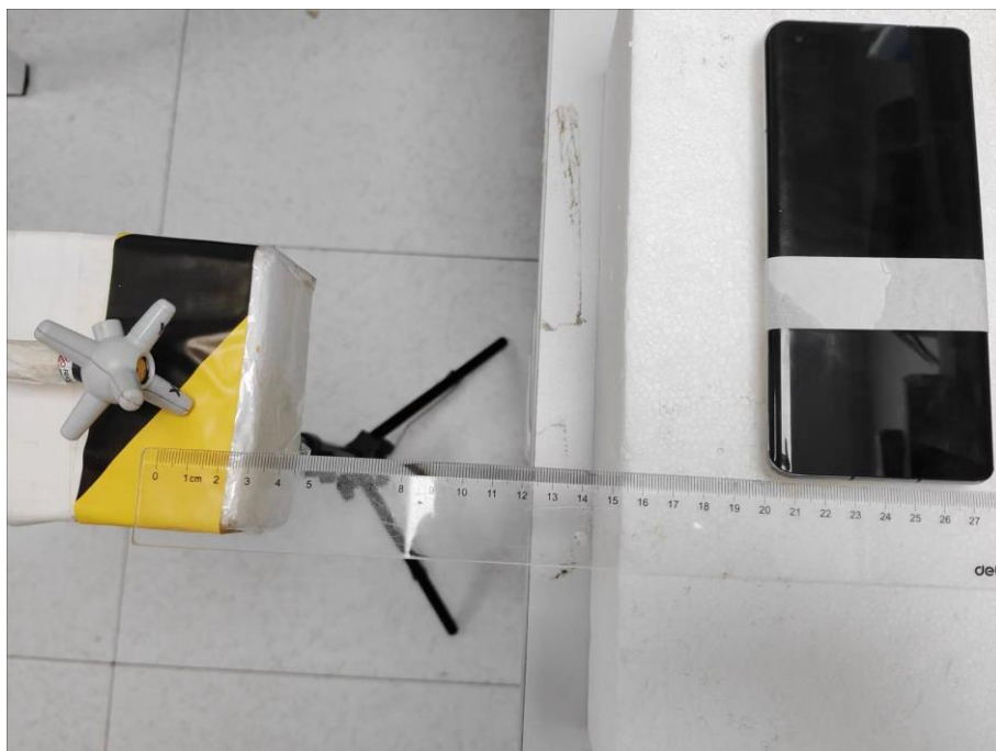
E-field Right Edge (20cm)
