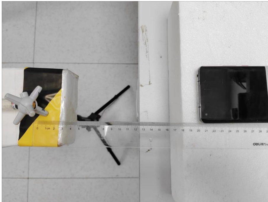
E-field Top Edge (20cm)
