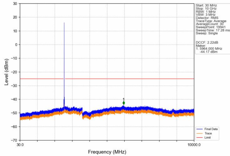
Band41 20MHz QPSK LCH 2565MHz RB 1 0 NTNV
