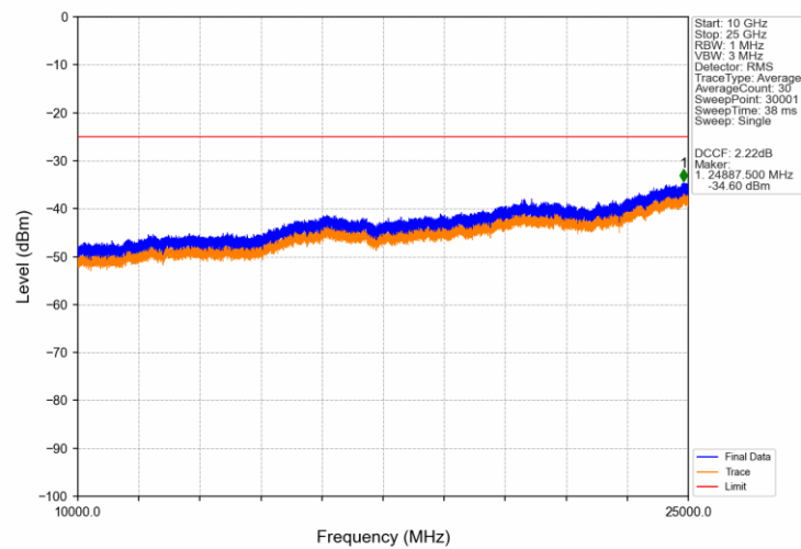
Band41 20MHz QPSK LCH 2565MHz RB 1 0 NTNV
