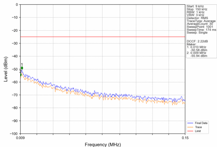
Band41_20MHz_QPSK_HCH_2645MHz_RB_1_0_NTNV
