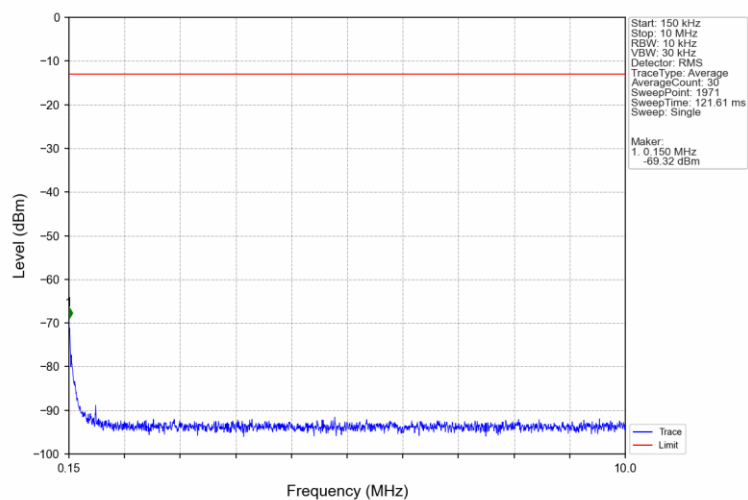
Band5 1.4MHz QPSK MCH 836.5MHz RB 1 0 NTV
