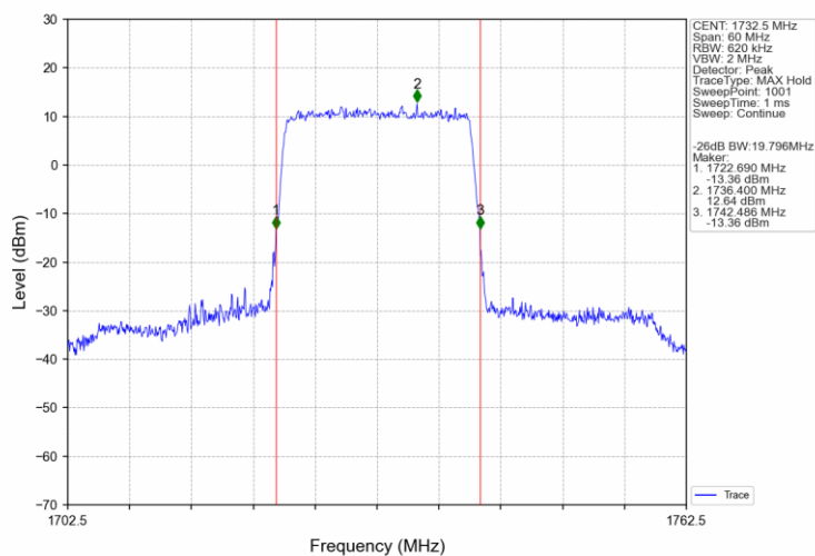
Band4 20MHz QPSK MCH 1732.5MHz RB 100 0 NTNV
