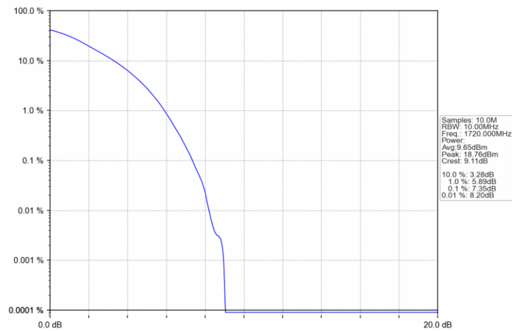
Band4 20MHz 16QAM LCH 1720MHz RB 27 0 NTV
