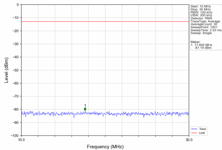
Band2 15MHz QPSK LCH 1857.5MHz RB 1 0 NTNV
