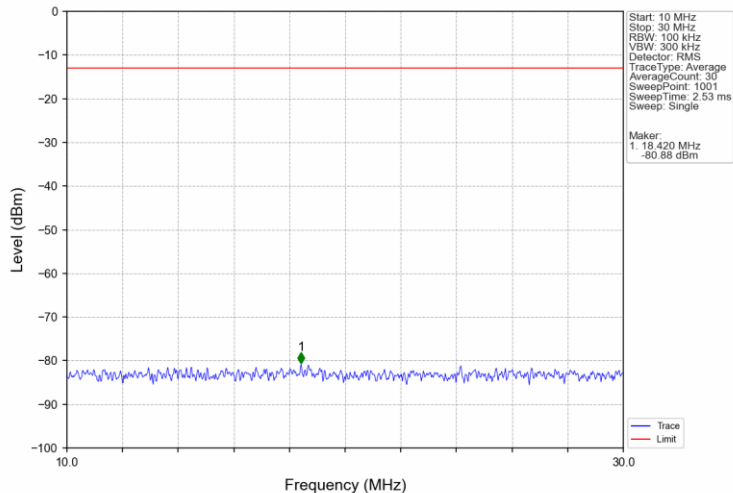
Band2_15MHz_QPSK_HCH_1902.5MHz_RB_1_0_NTNV
