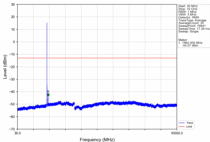
Band2_15MHz_QPSK_MCH_1880MHz_RB_1_0_NTNV
