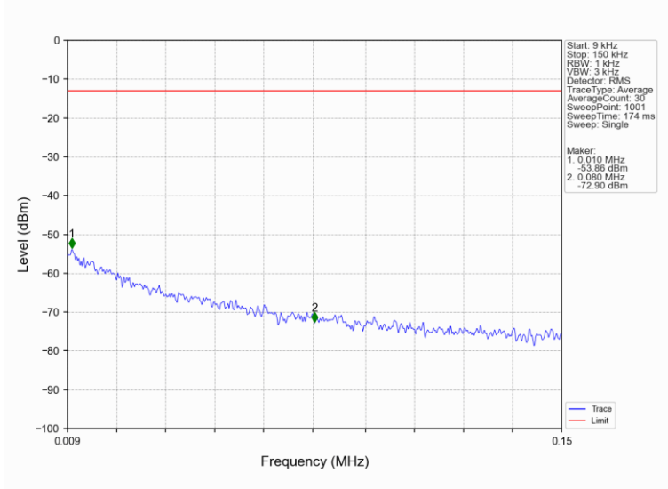
Band2_15MHz_QPSK_HCH_1902.5MHz_RB_1_0_NTNV
