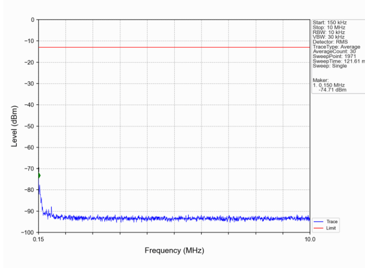
Band2_10MHz_QPSK_MCH_1880MHz_RB_1_0_NTNV
